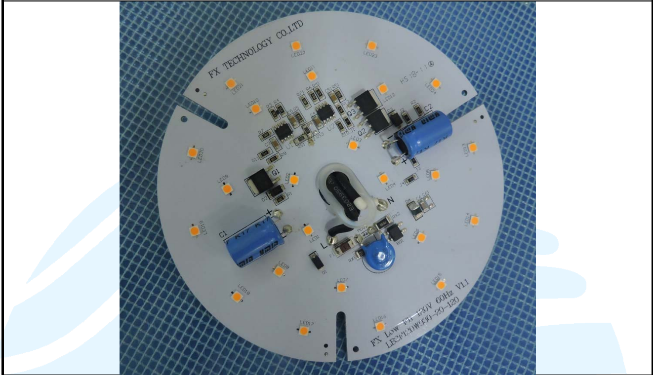
EUT Photo
