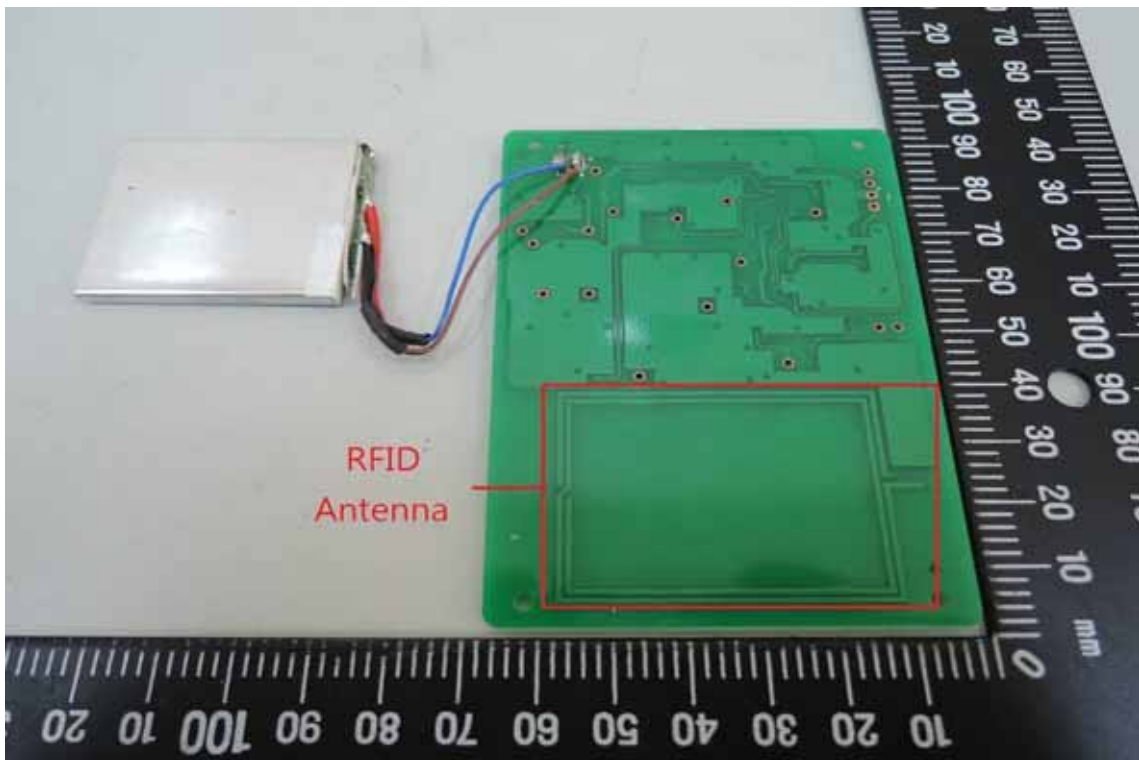
RFID Antenna
