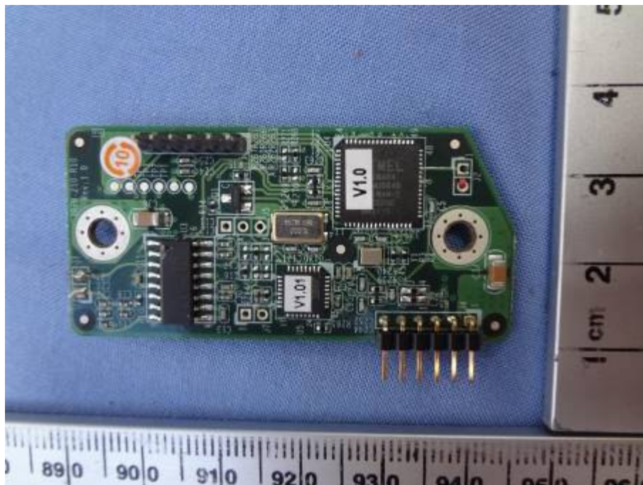
125KHz RFID Module PCB View 2
