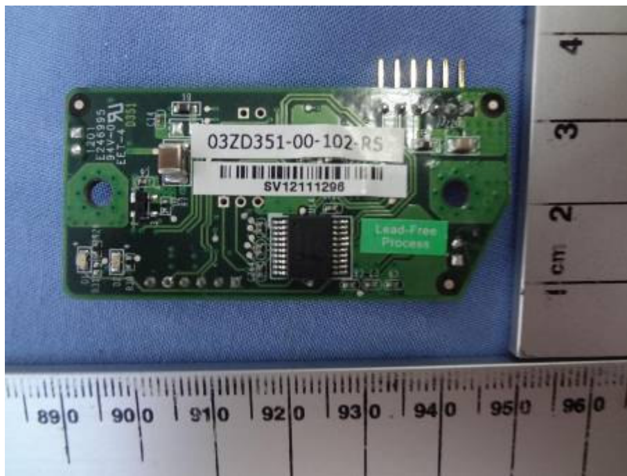
125KHz RFID Module PCB View 1
