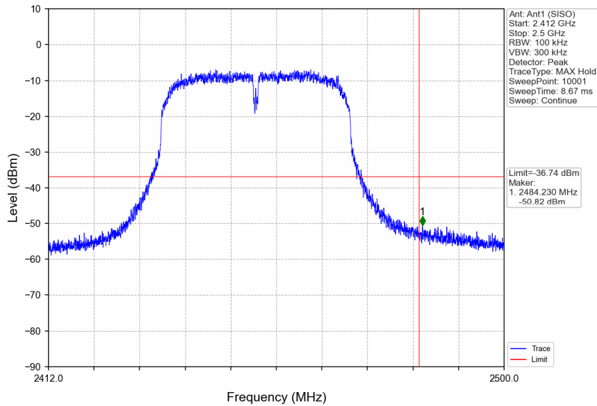
802.11n(HT40)_HCH_2452MHz_Ant1 (SISO)_NTNV
