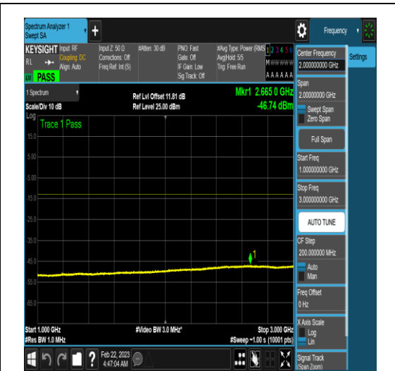
NTNV_N77-3450-3550_PC2_30_100_L_TID17_N /A_1000_3000_#1
