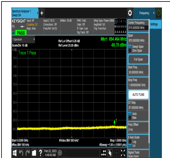
NTNV_N77-3450-3550_PC2_30_100_L_TID17_N /A_30_1000_#1
