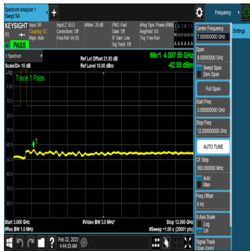
NTNV_N77-3450-3550_PC2_30_100_L_TID16_N /A_3000_12000_#1
