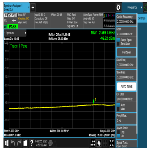
NTNV_N77-3450-3550_PC2_30_100_L_TID18_N /A_1000_3000_#1
