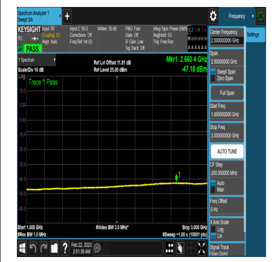
NTNV_N77-3450-3550_PC2_30_80_L_TID6_N/A _1000_3000_#1
