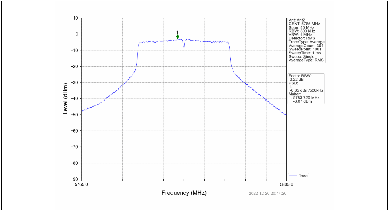
802.11n(HT20)_MCH_5785MHz_MIMO_NTNV
