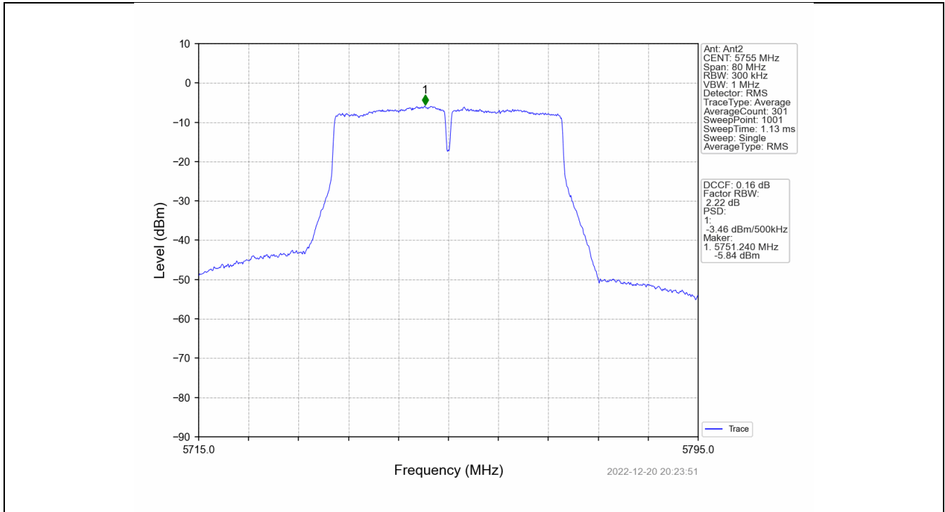
802.11n(HT40)_LCH_5755MHz_MIMO_NTNV
