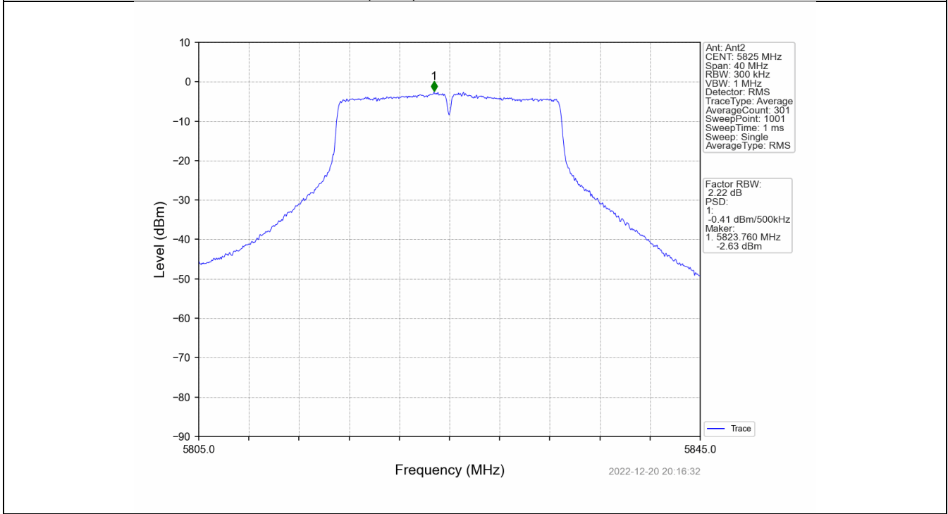
802.11n(HT20)_HCH_5825MHz_MIMO_NTNV
