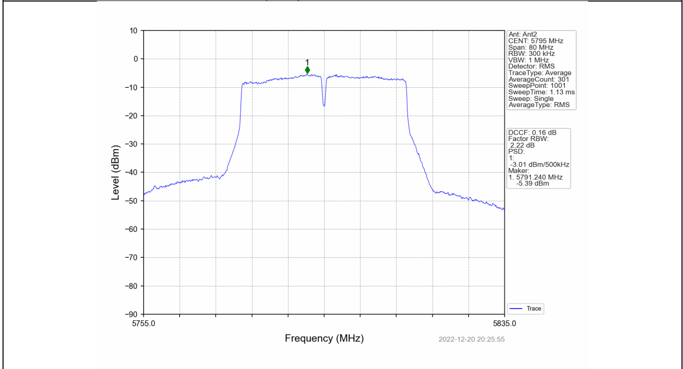
802.11n(HT40)_HCH_5795MHz_MIMO_NTNV
