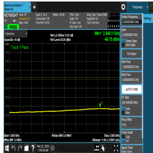
NTNV_N77-3450-3550_PC2_30_60_L_TID5_N/A _1000_3000_#1
