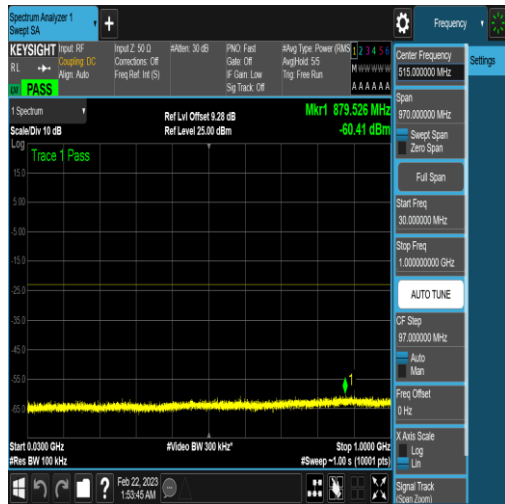
NTNV_N77-3450-3550_PC2_30_60_L_TID5_N/A _30_1000_#1
