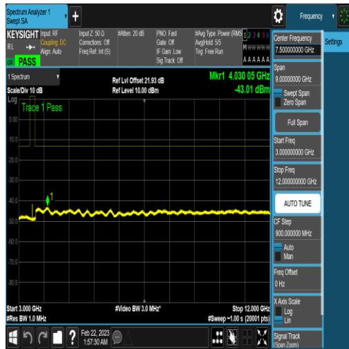
NTNV_N77-3450-3550_PC2_30_60_L_TID6_N/A _3000_12000_#1
