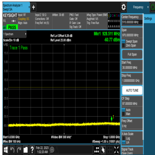
NTNV_N77-3450-3550_PC2_30_50_L_TID6_N/A _30_1000_#1
