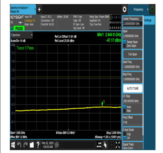
NTNV_N77-3450-3550_PC2_30_50_L_TID16_N/ A_1000_3000_#1
