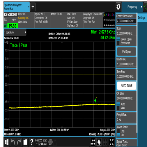
NTNV_N77-3450-3550_PC2_30_50_L_TID6_N/A _1000_3000_#1
