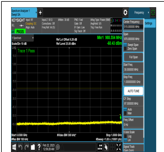
NTNV_N77-3450-3550_PC2_30_50_L_TID5_N/A _30_1000_#1
