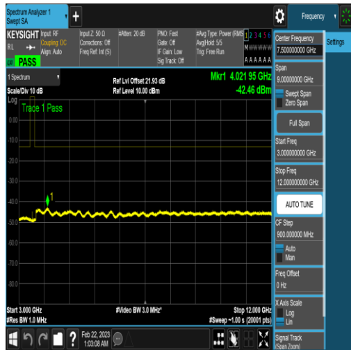
NTNV_N77-3450-3550_PC2_30_50_L_TID6_N/A _3000_12000_#1
