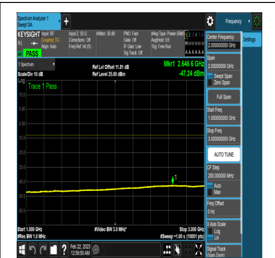
NTNV_N77-3450-3550_PC2_30_50_L_TID5_N/A _1000_3000_#1
