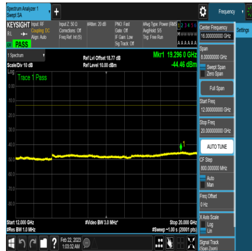
NTNV_N77-3450-3550_PC2_30_50_L_TID6_N/A _12000_20000_#1
