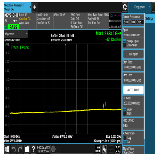
NTNV_N77-3450-3550_PC2_30_40_L_TID6_N/A _1000_3000_#1
