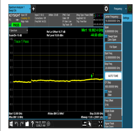
NTNV_N77-3450-3550_PC2_30_40_L_TID5_N/A _1000_3000_#1
