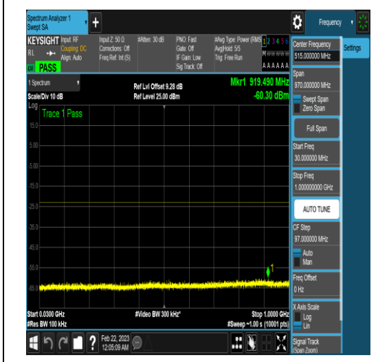
NTNV_N77-3450-3550_PC2_30_40_L_TID5_N/A _30_1000_#1
