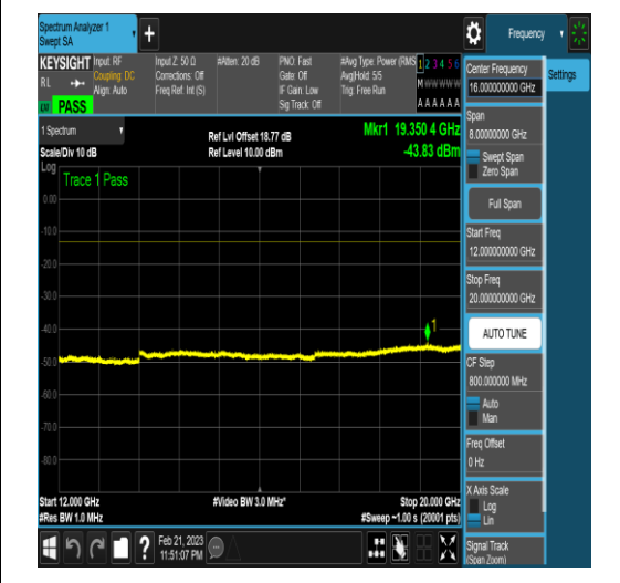
NTNV_N77-3450-3550_PC2_30_20_H_TID6_N/A _1000_3000_#1
