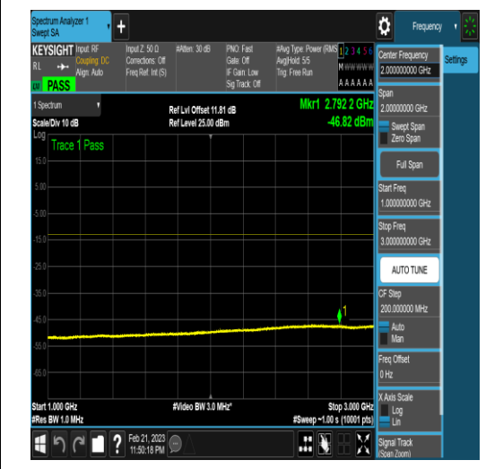
NTNV_N77-3450-3550_PC2_30_20_H_TID6_N/A _1000_3000_#1
