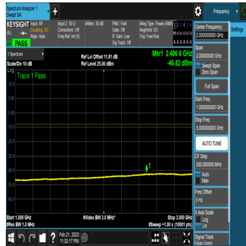
NTNV_N77-3450-3550_PC2_30_20_M_TID6_N/A _1000_3000_#1
