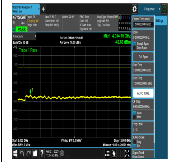
NTNV_N77-3450-3550_PC2_30_20_L_TID6_N/A _3000_12000_#1
