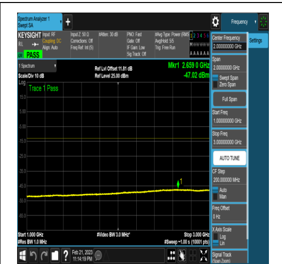
NTNV_N77-3450-3550_PC2_30_20_L_TID6_N/A _1000_3000_#1
