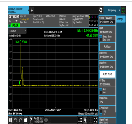
NTNV_N77-3450-3550_PC2_30_40_L_TID6_RID
