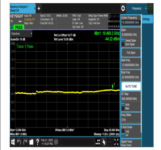
NTNV_N77-3450-3550_PC2_30_20_L_TID6_N/A _12000_20000_#1
