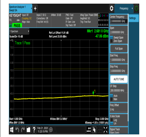
NTNV_N77-3450-3550_PC2_30_20_L_TID17_N/ A_1000_3000_#1
