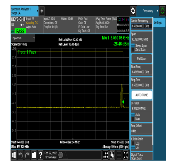
NTNV_N77-3450-3550_PC2_30_80_L_TID6_RID
