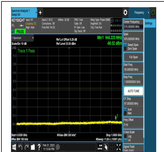
NTNV_N77-3450-3550_PC2_30_20_L_TID6_N/A _30_1000_#1
