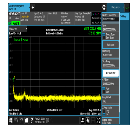
NTNV_N77-3450-3550_PC2_30_20_L_TID6_N/A _12000_20000_#1
