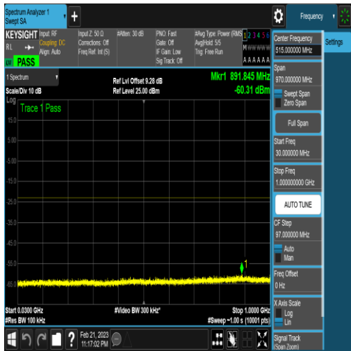
NTNV_N77-3450-3550_PC2_30_20_L_TID16_N/ A_30_1000_#1
