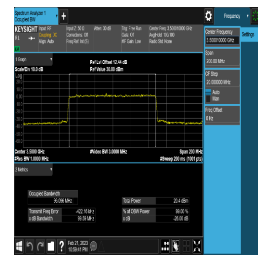
NTNV_N77-3450-3550_PC2_30_100_L_TID5_An
