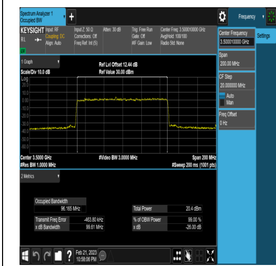
NTNV_N77-3450-3550_PC2_30_100_L_TID1_An
