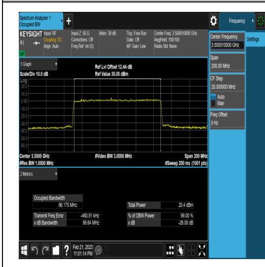
NTNV_N77-3450-3550_PC2_30_100_L_TID1_An
