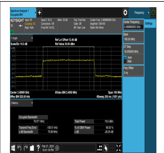
NTNV_N77-3450-3550_PC2_30_80_L_TID5_Ant
