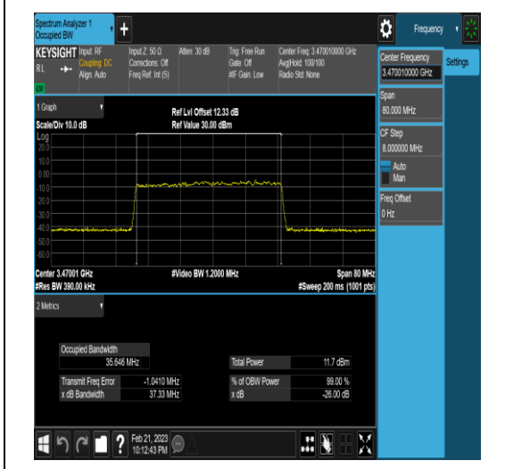
NTNV_N77-3450-3550_PC2_30_40_L_TID1_Ant
