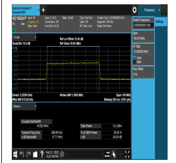
NTNV_N77-3450-3550_PC2_30_50_H_TID1_Ant
