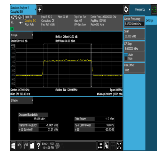
NTNV_N77-3450-3550_PC2_30_40_L_TID5_Ant
