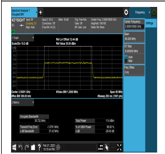
NTNV_N77-3450-3550_PC2_30_40_L_TID1_Ant
