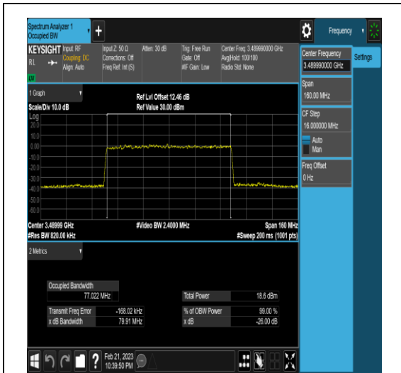
NTNV_N77-3450-3550_PC2_30_80_L_TID1_Ant
