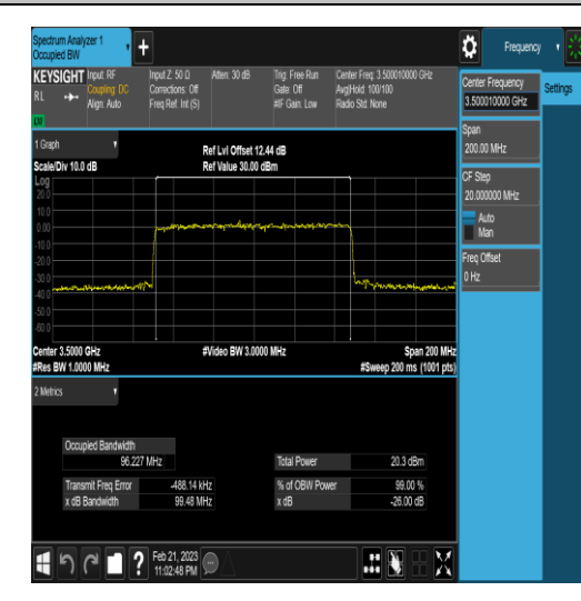
NTNV_N77-3450-3550_PC2_30_100_L_TID5_An
