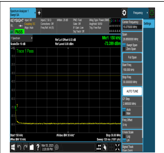
NTNV_N78-3700-3800_PC2_30_100_L_TID5_N/ A_0.15_30_#1
