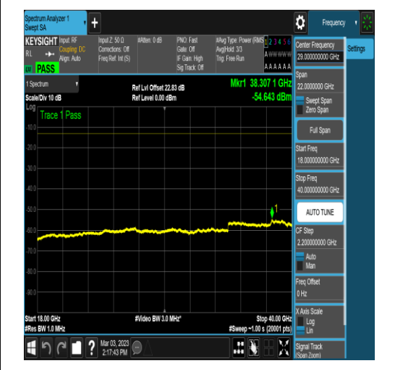
NTNV_N78-3700-3800_PC2_30_90_H_TID18_N/ A_18000_40000_#1
