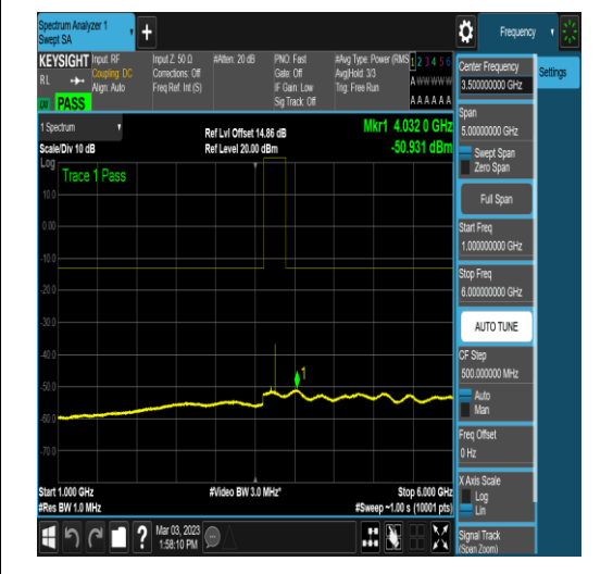
NTNV_N78-3700-3800_PC2_30_90_M_TID16_N/ A_1000_6000_#1
