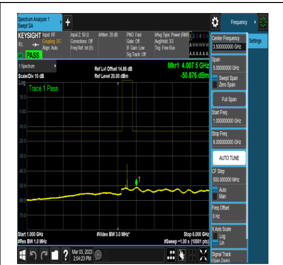
NTNV_N78-3700-3800_PC2_30_90_H_TID4_N/A _1000_6000_#1
