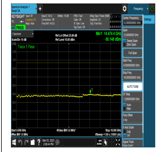
NTNV_N78-3700-3800_PC2_30_90_H_TID6_N/A _30_1000_#1
