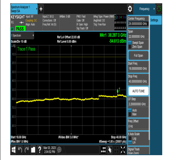
NTNV_N78-3700-3800_PC2_30_90_H_TID4_N/A _18000_40000_#1
