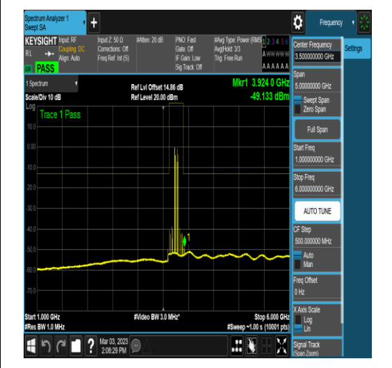
NTNV_N78-3700-3800_PC2_30_90_H_TID6_N/A _1000_6000_#1
