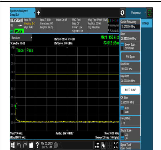
NTNV_N78-3700-3800_PC2_30_90_H_TID6_N/A _0.15_30_#1
