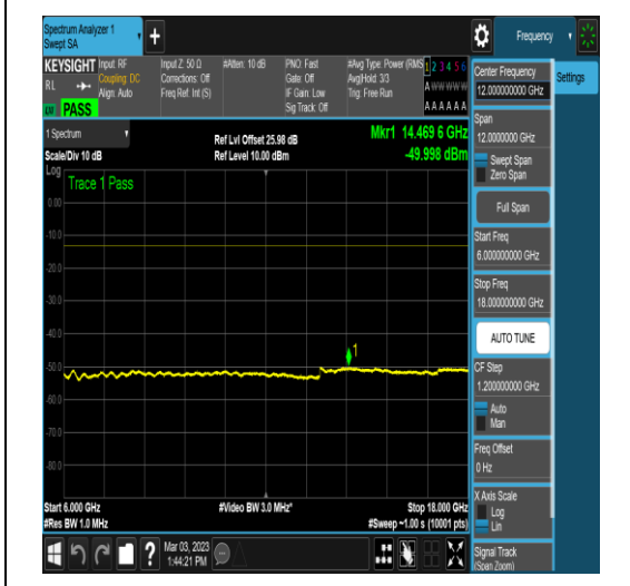
NTNV_N78-3700-3800_PC2_30_90_L_TID6_N/A _6000_18000_#1
