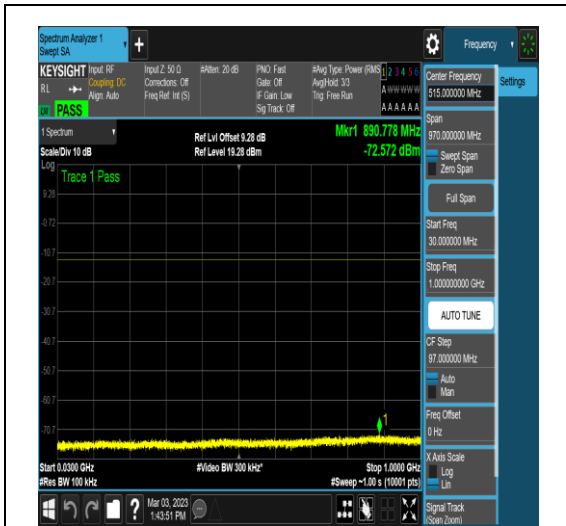
NTNV_N78-3700-3800_PC2_30_90_L_TID6_N/A _30_1000_#1
