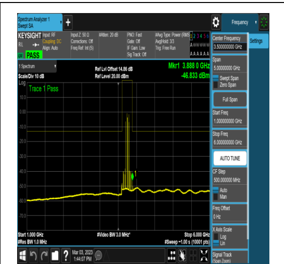
NTNV_N78-3700-3800_PC2_30_90_L_TID6_N/A _1000_6000_#1
