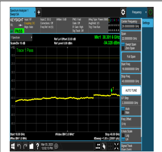
NTNV_N78-3700-3800_PC2_30_50_L_TID17_N/A_18000_40000_#1
