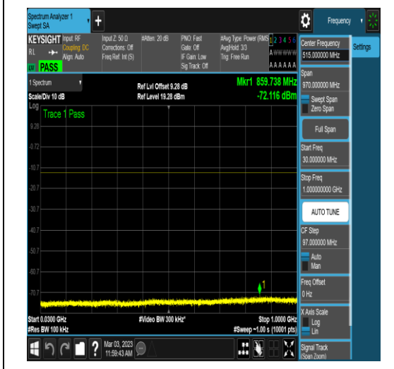
NTNV_N78-3700-3800_PC2_30_50_L_TID16_N/ A_30_1000_#1
