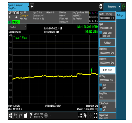
NTNV_N78-3700-3800_PC2_30_50_L_TID16_N/ A_1000_6000_#1
