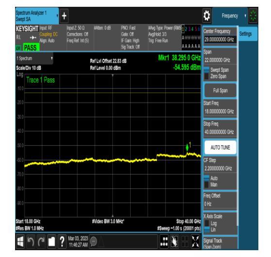
NTNV_N78-3700-3800_PC2_30_40_H_TID6_N/A _18000_40000_#1
