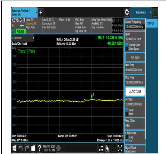
NTNV_N78-3700-3800_PC2_30_50_L_TID17_N/A_6000_18000_#1
