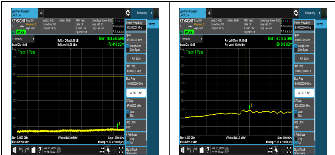
NTNV_N78-3700-3800_PC2_30_50_L_TID5_N/A _30_1000_#1 NTNV_N78-3700-3800_PC2_30_50_L_TID5_N/A _1000_6000_#1
