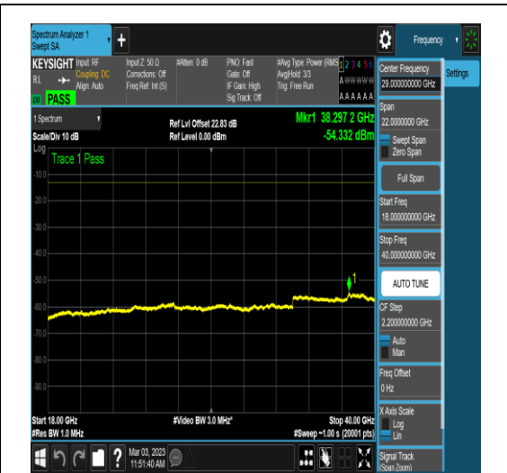
NTNV_N78-3700-3800_PC2_30_40_H_TID18_N/A_18000_40000_#1
