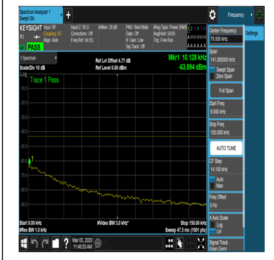
NTNV_N78-3700-3800_PC2_30_40_H_TID6_N/A _6000_18000_#1
