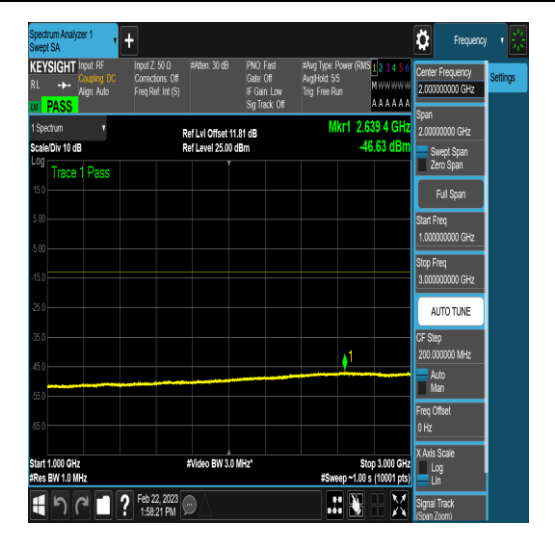
NTNV_N78-3650-3700_PC2_30_40_H_TID16_N/ A_1000_3000_#1
