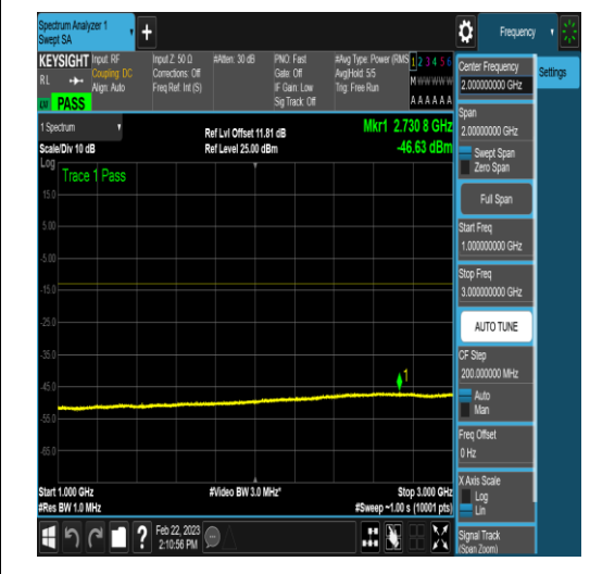
NTNV_N78-3650-3700_PC2_30_50_M_TID16_N/ A_1000_3000_#1
