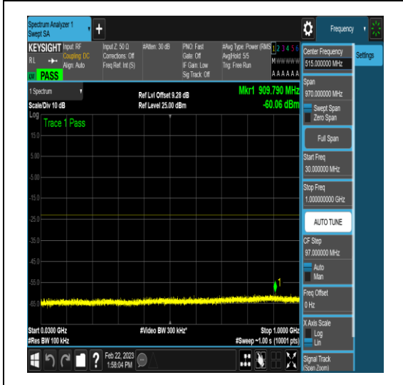
NTNV_N78-3650-3700_PC2_30_40_H_TID16_N/ A_30_1000_#1
