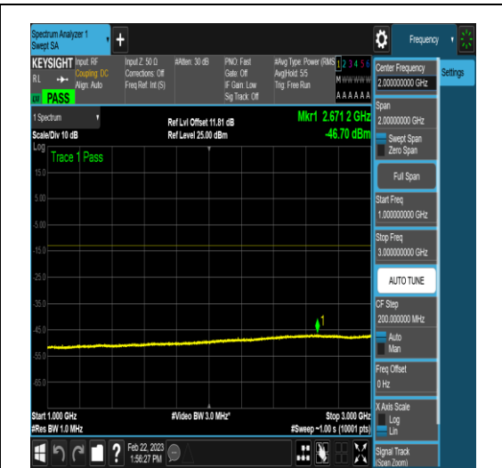
NTNV_N78-3650-3700_PC2_30_40_H_TID6_N/A _1000_3000_#1
