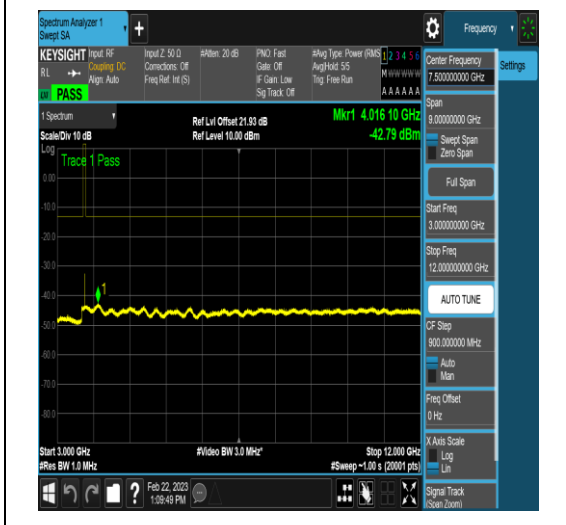
NTNV_N78-3650-3700_PC2_30_20_M_TID16_N/ A_30_1000_#1
