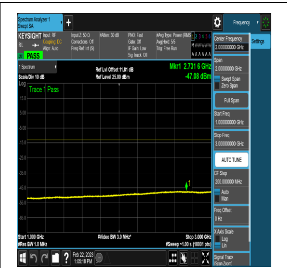
NTNV_N78-3650-3700_PC2_30_20_M_TID5_N/A _1000_3000_#1
