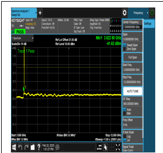
NTNV_N78-3650-3700_PC2_30_20_L_TID18_N/A_3000_12000_#1
