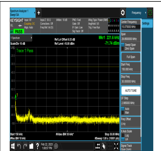
NTNV_N78-3650-3700_PC2_30_20_M_TID16_N/ A_0.15_30_#1
