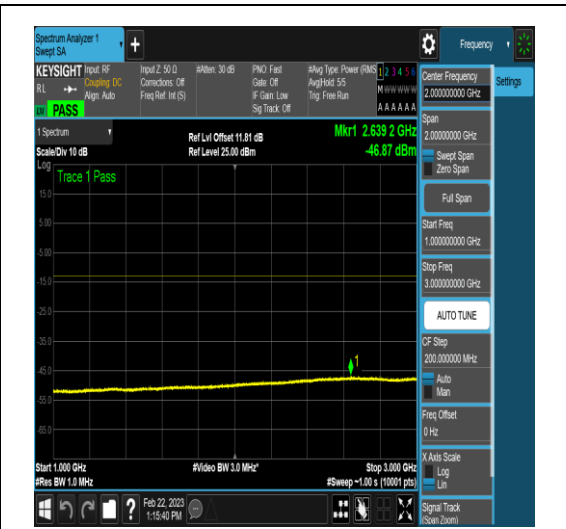
NTNV_N78-3650-3700_PC2_30_20_H_TID4_N/A _1000_3000_#1
