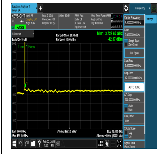
NTNV_N78-3650-3700_PC2_30_20_H_TID6_N/A _30_1000_#1
