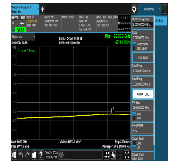
NTNV_N78-3650-3700_PC2_30_20_M_TID16_N/ A_1000_3000_#1
