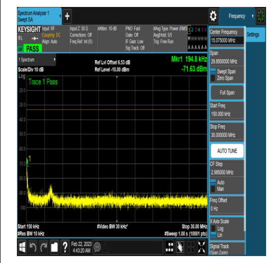
NTNV_N78-3450-3550_PC2_30_100_L_TID16_N /A_0.15_30_#1
