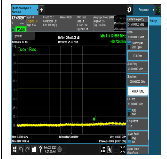
NTNV_N78-3450-3550_PC2_30_100_L_TID5_N/ A_30_1000_#1
