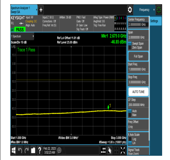
NTNV_N78-3450-3550_PC2_30_90_L_TID17_N/ A_1000_3000_#1
