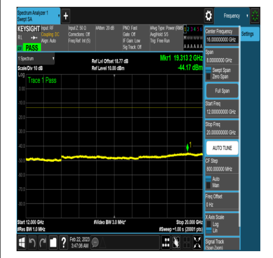
NTNV_N78-3450-3550_PC2_30_90_L_TID6_N/A _12000_20000_#1
