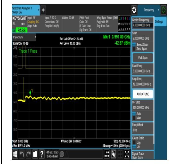
NTNV_N78-3450-3550_PC2_30_90_L_TID6_N/A _3000_12000_#1
