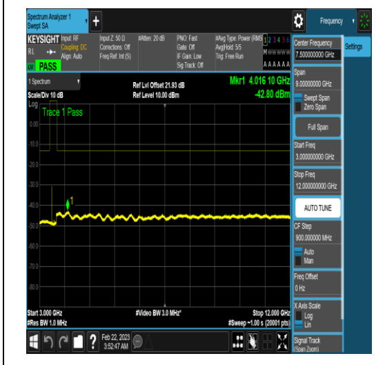
NTNV_N78-3450-3550_PC2_30_90_L_TID17_N/ A_30_1000_#1
