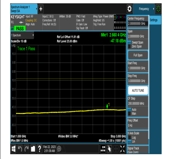
NTNV_N78-3450-3550_PC2_30_80_L_TID6_N/A _1000_3000_#1
