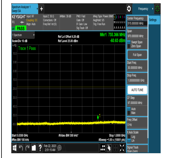
NTNV_N78-3450-3550_PC2_30_80_L_TID6_N/A _30_1000_#1
