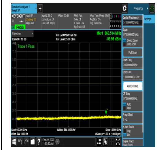
NTNV_N78-3450-3550_PC2_30_60_L_TID4_N/A _30_1000_#1
