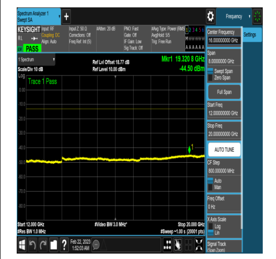
NTNV_N78-3450-3550_PC2_30_60_L_TID4_N/A _1000_3000_#1
