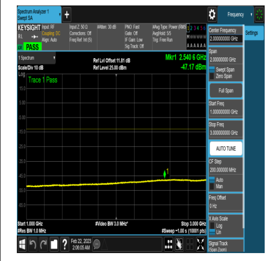
NTNV_N78-3450-3550_PC2_30_60_L_TID18_N/ A_1000_3000_#1
