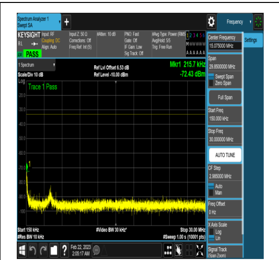
NTNV_N78-3450-3550_PC2_30_60_L_TID18_N/ A_0.15_30_#1
