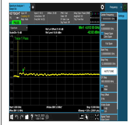
NTNV_N78-3450-3550_PC2_30_50_L_TID16_N/ A_30_1000_#1
