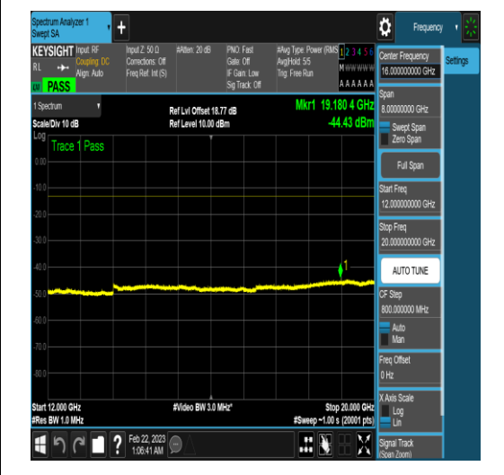
NTNV_N78-3450-3550_PC2_30_50_L_TID16_N/ A_1000_3000_#1
