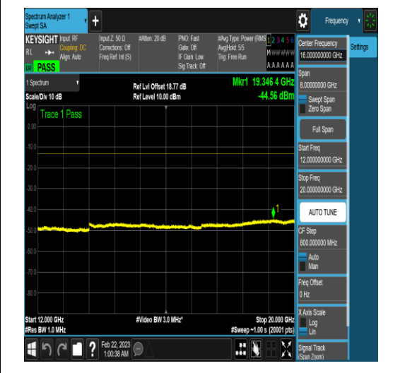
NTNV_N78-3450-3550_PC2_30_50_L_TID5_N/A _12000_20000_#1
