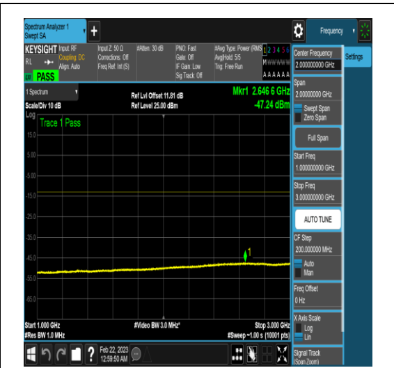
NTNV_N78-3450-3550_PC2_30_50_L_TID5_N/A _1000_3000_#1
