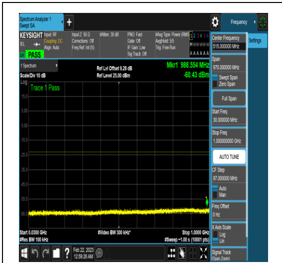
NTNV_N78-3450-3550_PC2_30_50_L_TID5_N/A _30_1000_#1
