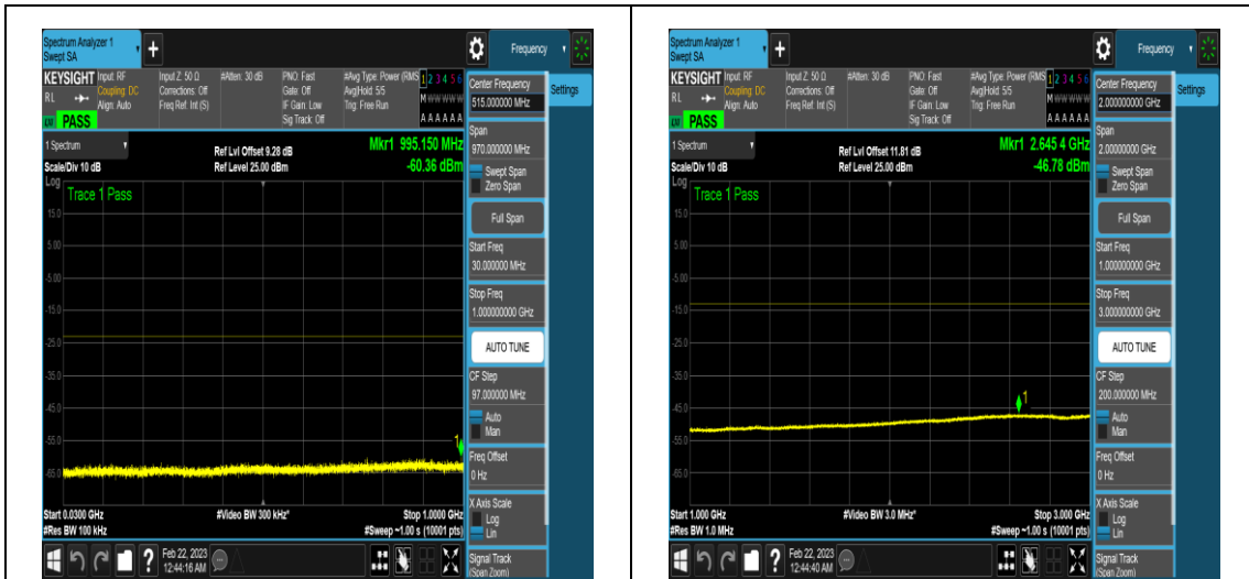
NTNV_N78-3450-3550_PC2_30_40_H_TID6_N/A _30_1000_#1
