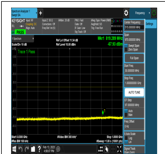
NTNV_N41_PC2_30_100_M_TID21_N/A_30_100 0_#1
