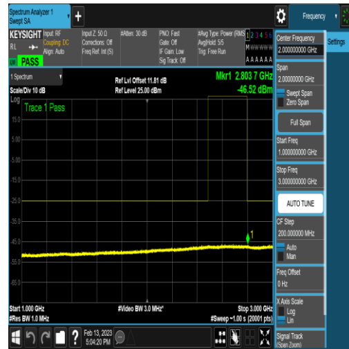
NTNV_N41_PC2_30_100_H_TID6_N/A_1000_30 00_#1
