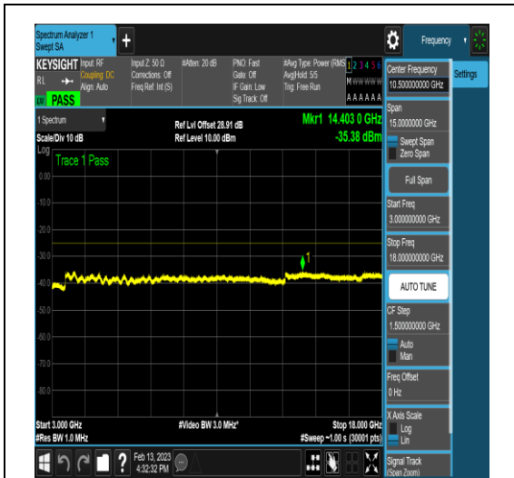
NTNV_N41_PC2_30_100_L_TID9_N/A_3000_18000_#1
