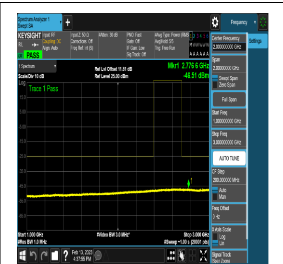
NTNV_N41_PC2_30_100_L_TID18_N/A_1000_3 000_#1
