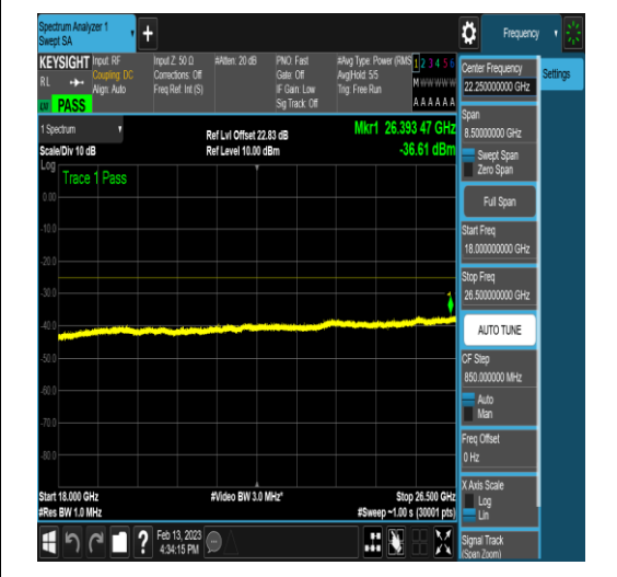
NTNV_N41_PC2_30_100_L_TID12_N/A_1000_3000_#1
