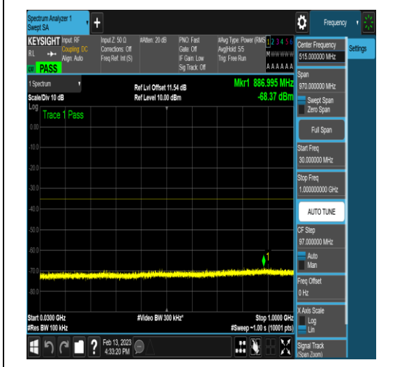
NTNV_N41_PC2_30_100_L_TID12_N/A_30_1000_#1
