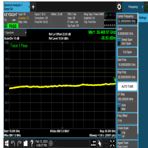
NTNV_N41_PC2_30_60_M_TID24_N/A_18000_2 6500_#1
