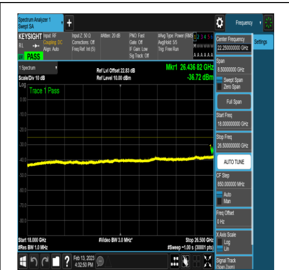
NTNV_N41_PC2_30_100_L_TID9_N/A_18000_26500_#1
