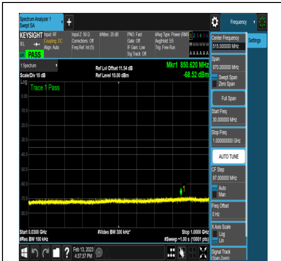
NTNV_N41_PC2_30_100_L_TID18_N/A_30_100 0_#1
