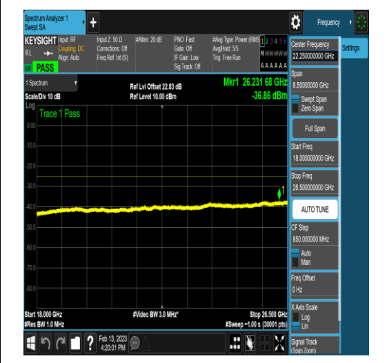
NTNV_N41_PC2_30_60_H_TID15_N/A_18000_26500_#1
