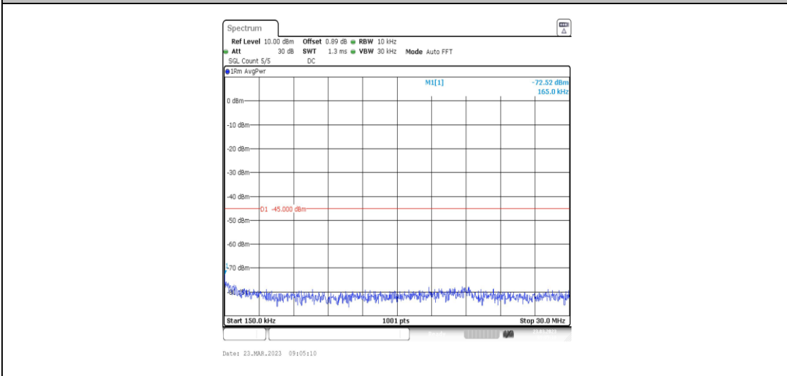
38-38-20MHz-20MHz-QPSK-QPSK-37952-38150-1RB#99-0RB#0-0.15~30MHz
