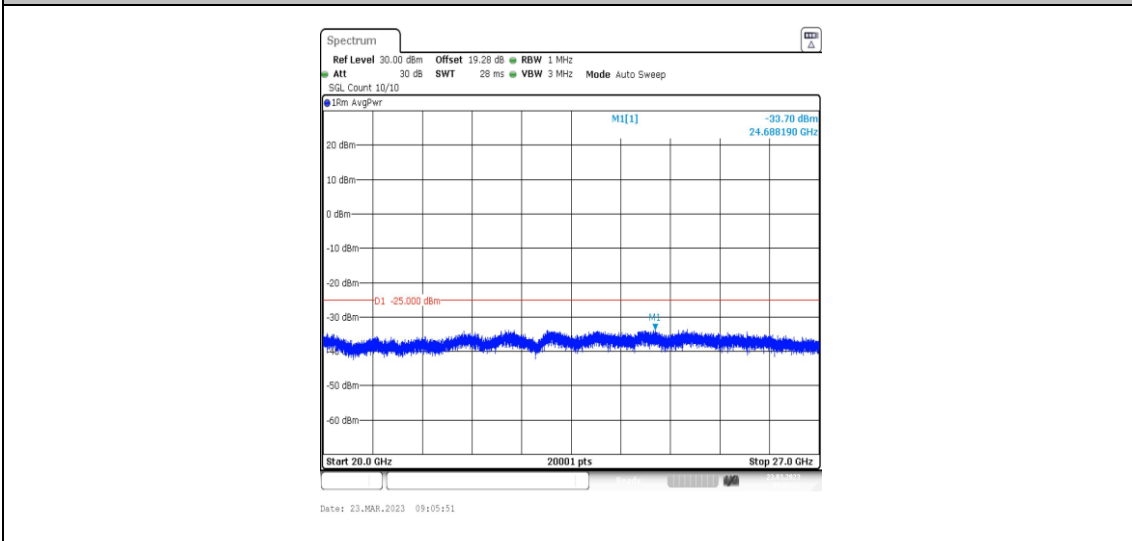
38-38-20MHz-20MHz-QPSK-QPSK-37952-38150-1RB#99-ORB#0-20000~27000MHz
