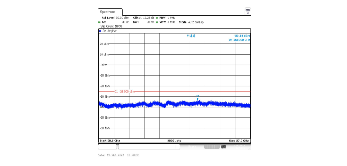
38-38-20MHz-20MHz-16QAM-16QAM-37901-38099-1RB#99-0RB#0-20000~27000MHz
