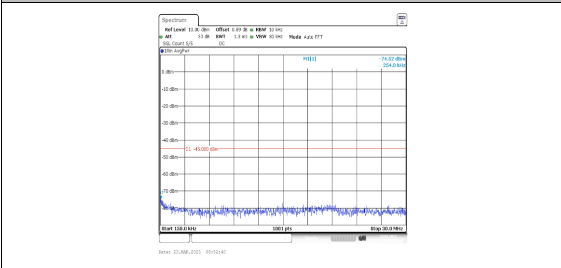
38-38-20MHz-20MHz-QPSK-QPSK-37901-38099-1RB#0-1RB#99-0.15~30MHz
