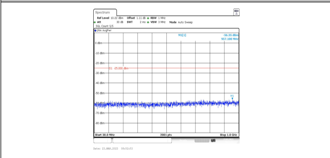
38-38-20MHz-20MHz-QPSK-QPSK-37901-38099-1RB#0-1RB#99-30~1000MHz
