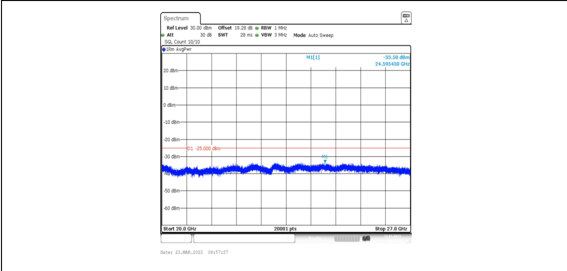
38-38-20MHz-20MHz-QPSK-QPSK-37901-38099-100RB#0-100RB#0-20000~27000MHz
