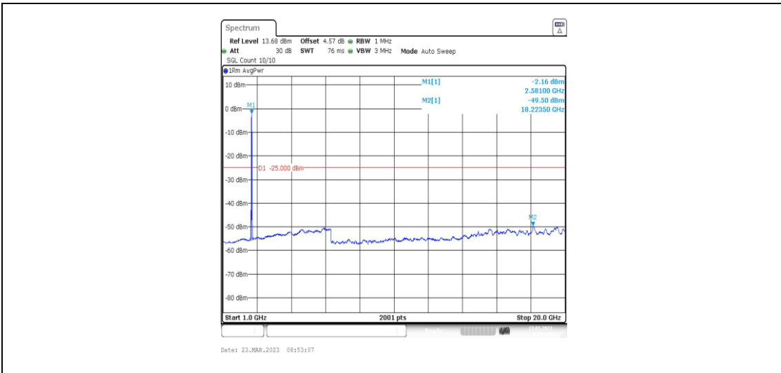
38-38-20MHz-20MHz-QPSK-QPSK-37901-38099-1RB#0-1RB#99-1000~20000MHz
