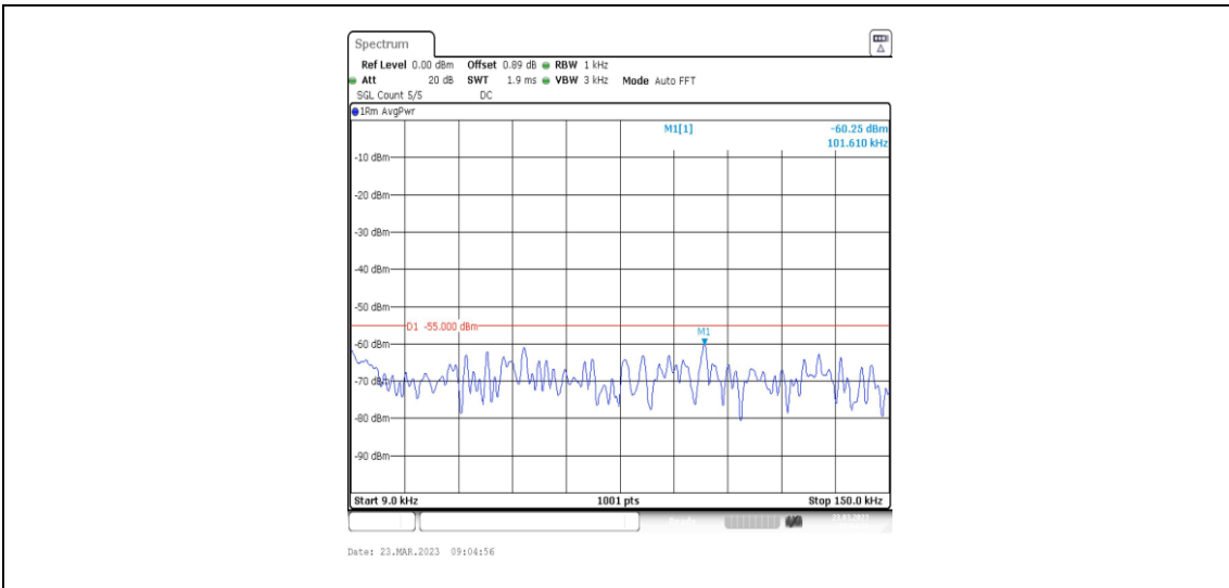
38-38-20MHz-20MHz-QPSK-QPSK-37952-38150-1RB#99-0RB#0-0.009~0.15MHz
