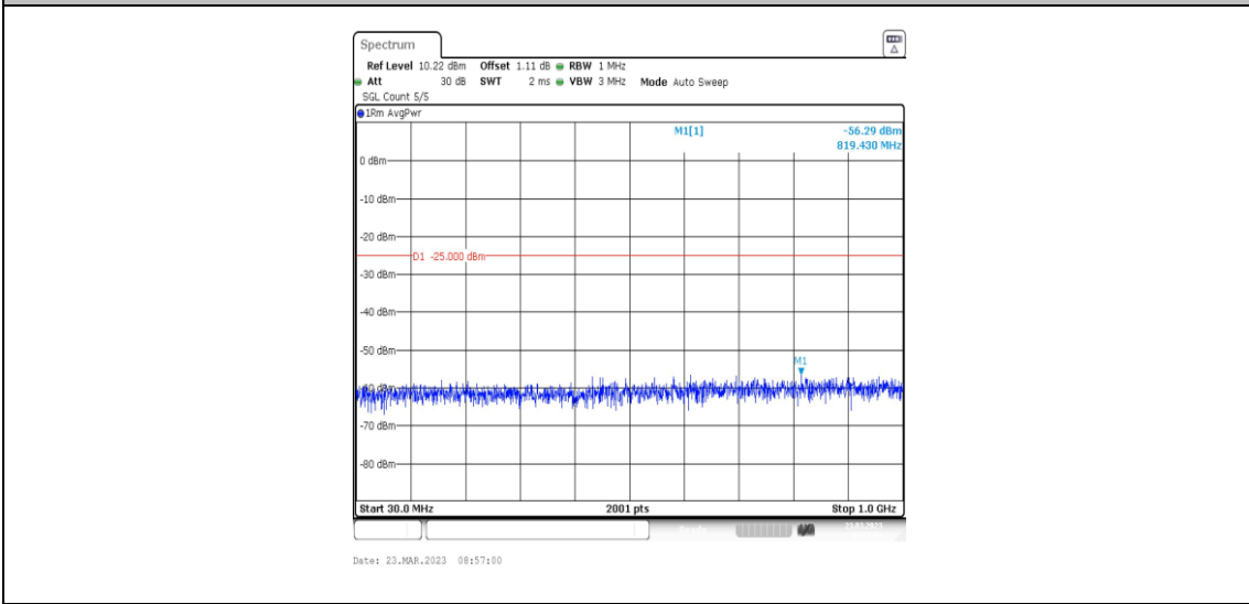
38-38-20MHz-20MHz-QPSK-QPSK-37901-38099-100RB#0-100RB#0-30~1000MHz
