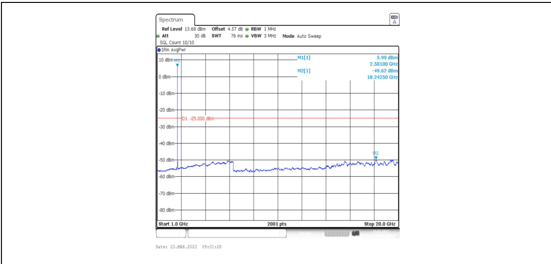
38-38-20MHz-20MHz-QPSK-QPSK-37952-38150-1RB#0-0RB#0-1000~20000MHz
