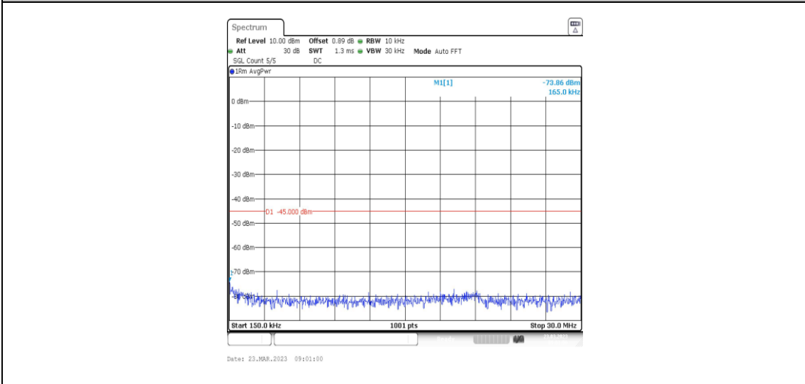
38-38-20MHz-20MHz-QPSK-QPSK-37952-38150-1RB#0-ORB#0-0.15~30MHz
