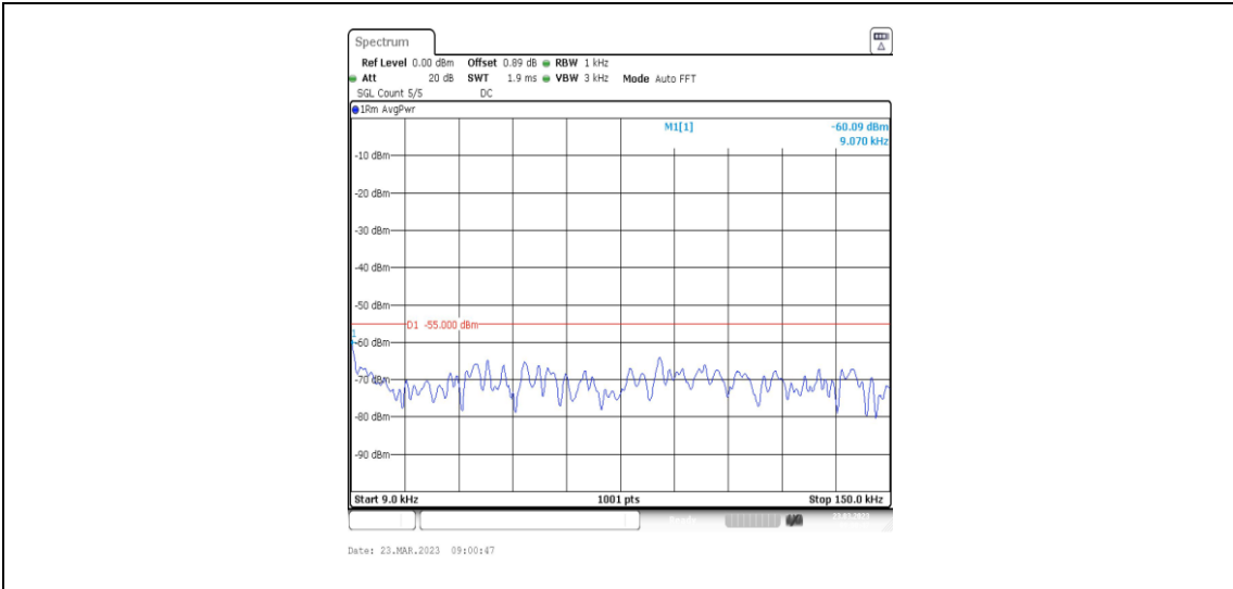
38-38-20MHz-20MHz-QPSK-QPSK-37952-38150-1RB#0-ORB#0-0.009~0.15MHz
