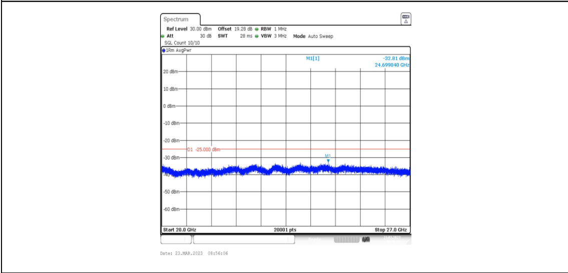
38-38-20MHz-20MHz-64QAM-64QAM-37901-38099-1RB#0-1RB#99-20000~27000MHz
