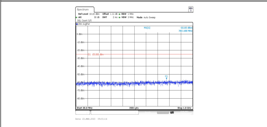
38-38-20MHz-20MHz-QPSK-QPSK-37952-38150-1RB#0-ORB#0-30~1000MHz
