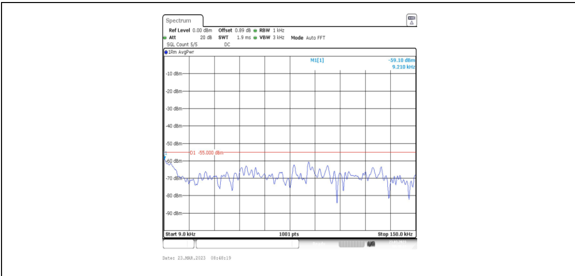
38-38-20MHz-20MHz-QPSK-QPSK-37901-38099-1RB#99-0RB#0-0.009~0.15MHz
