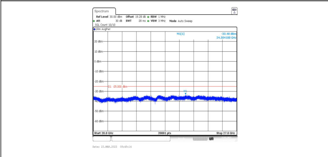
38-38-20MHz-20MHz-QPSK-QPSK-37901-38099-1RB#99-ORB#0-20000~27000MHz
