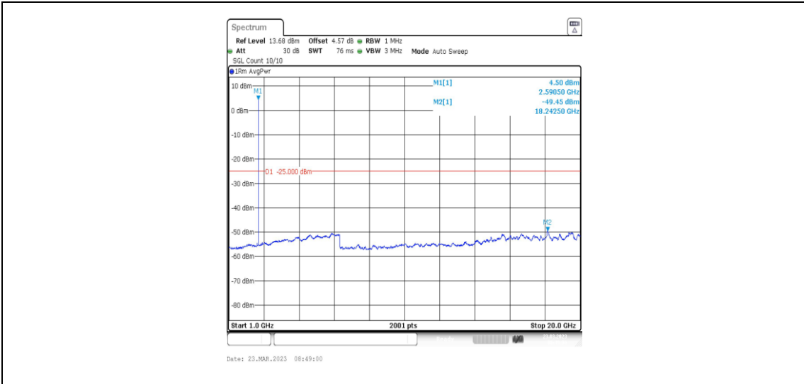
38-38-20MHz-20MHz-QPSK-QPSK-37901-38099-1RB#99-ORB#0-1000~20000MHz
