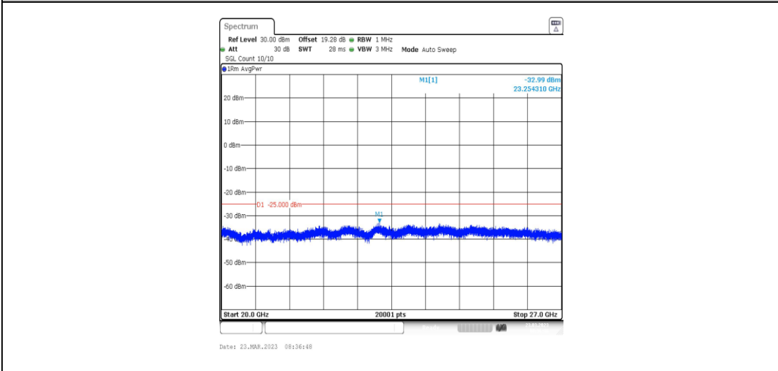
38-38-20MHz-20MHz-QPSK-QPSK-37850-38048-1RB#0-1RB#99-20000~27000MHz
