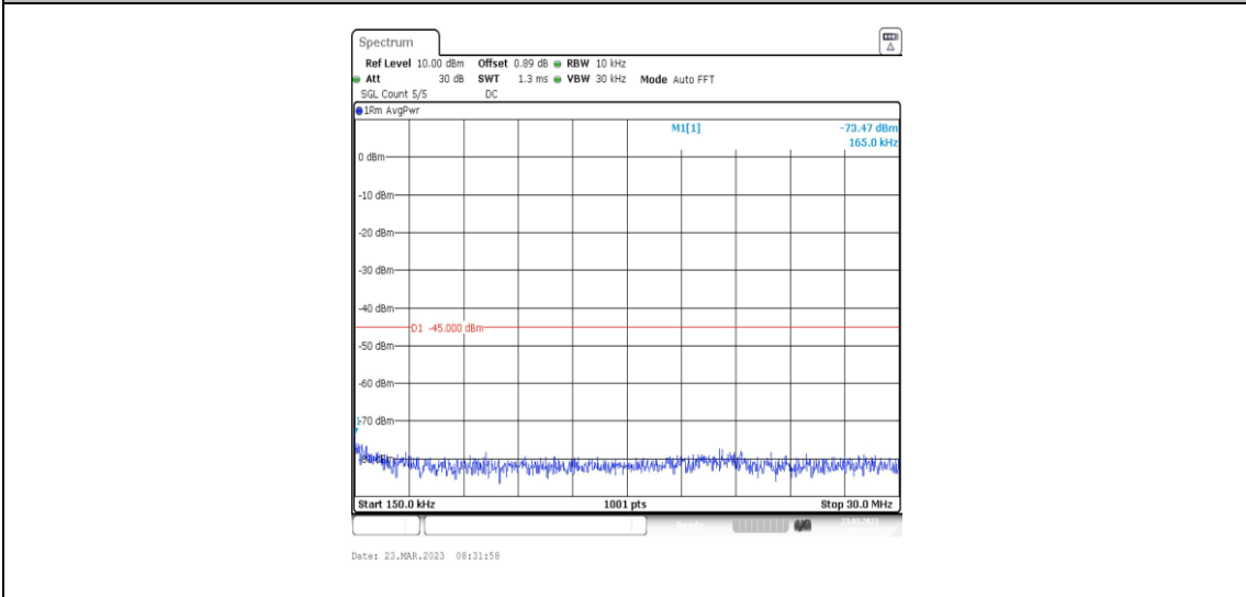
38-38-20MHz-20MHz-QPSK-QPSK-37850-38048-1RB#99-0RB#0-0.15~30MHz
