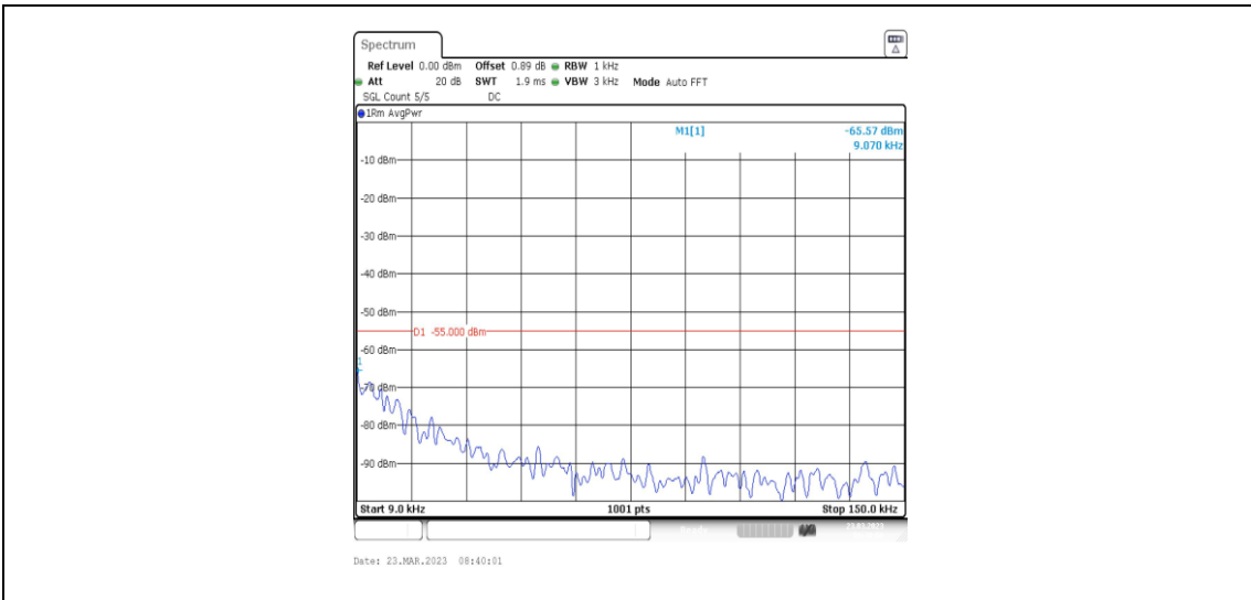
38-38-20MHz-20MHz-QPSK-QPSK-37850-38048-100RB#0-100RB#0-0.009~0.15MHz
