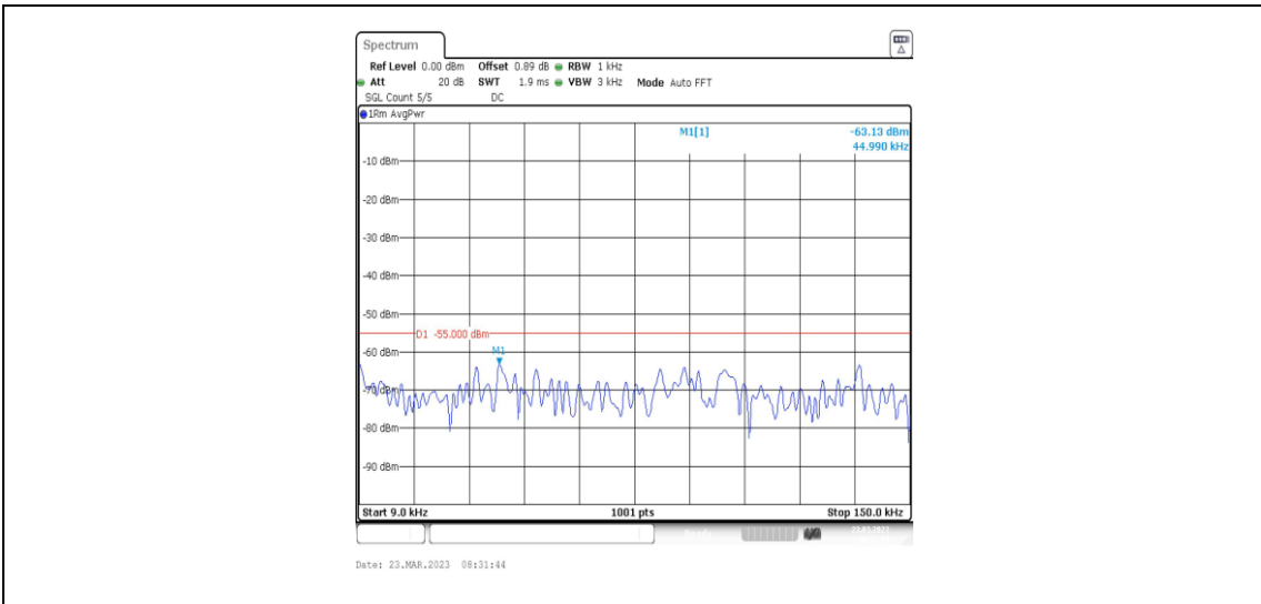
38-38-20MHz-20MHz-QPSK-QPSK-37850-38048-1RB#99-0RB#0-0.009~0.15MHz
