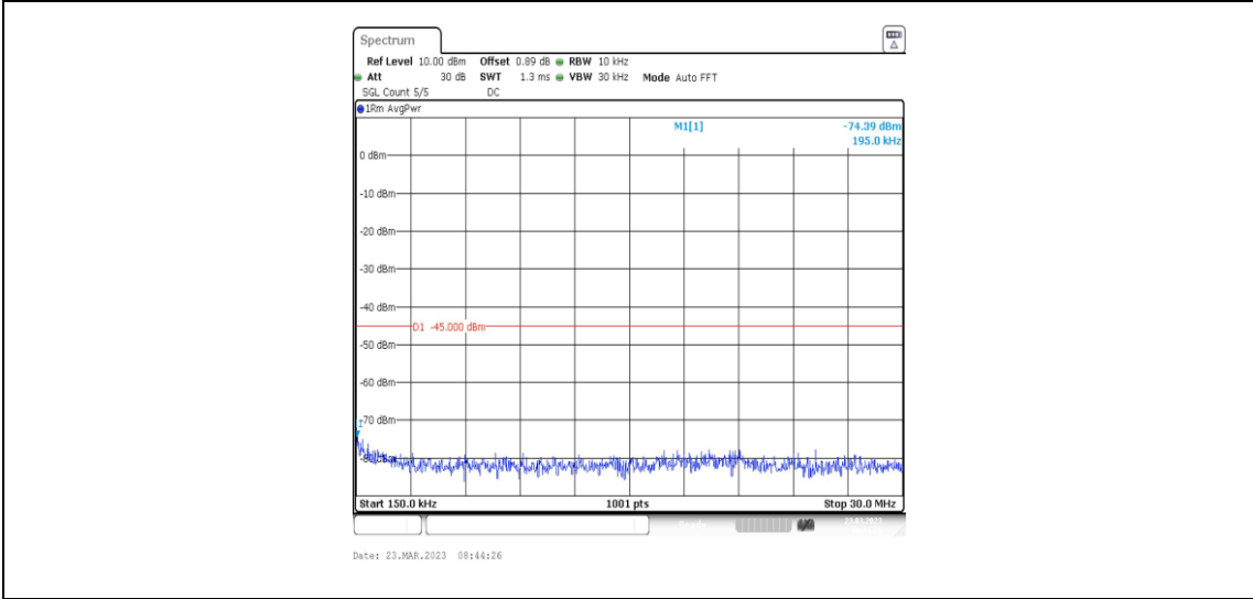
38-38-20MHz-20MHz-QPSK-QPSK-37901-38099-1RB#0-0RB#0-0.15~30MHz
