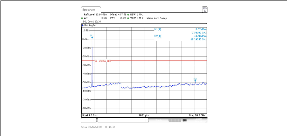
38-38-20MHz-20MHz-QPSK-QPSK-37850-38048-100RB#0-100RB#0-1000~20000MHz
