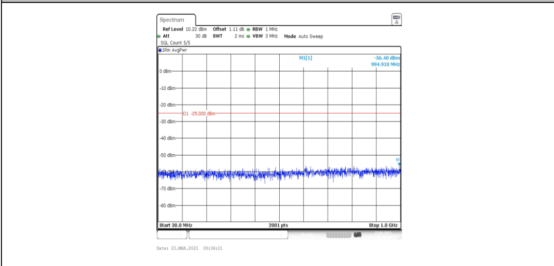
38-38-20MHz-20MHz-QPSK-QPSK-37850-38048-1RB#0-1RB#99-30~1000MHz
