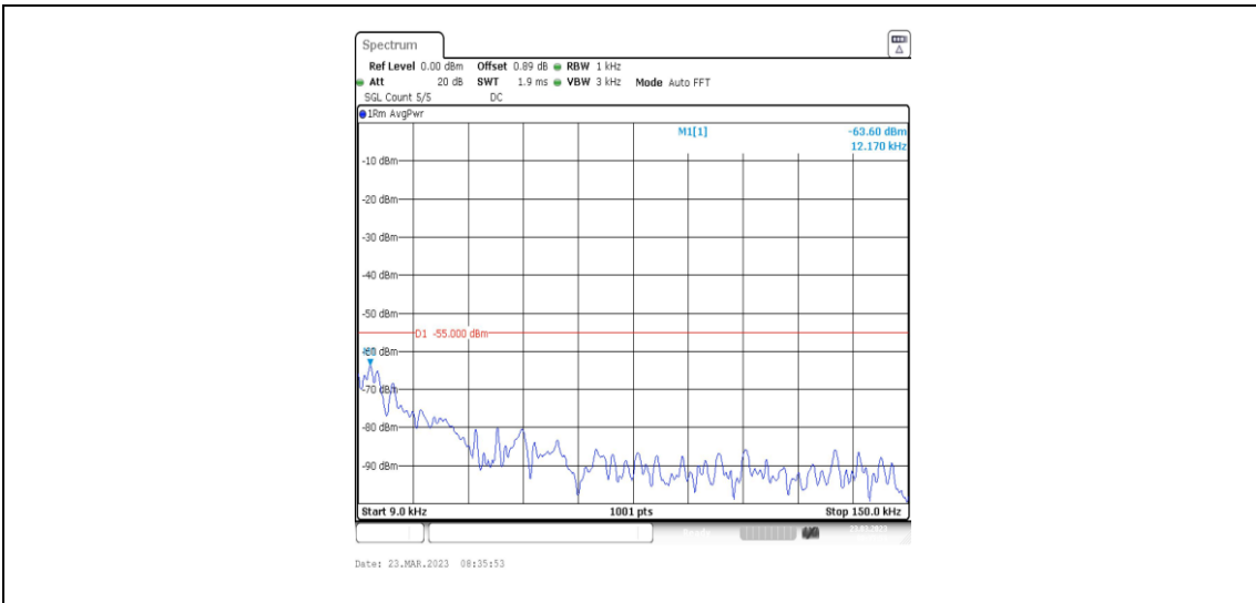
38-38-20MHz-20MHz-QPSK-QPSK-37850-38048-1RB#0-1RB#99-0.009~0.15MHz
