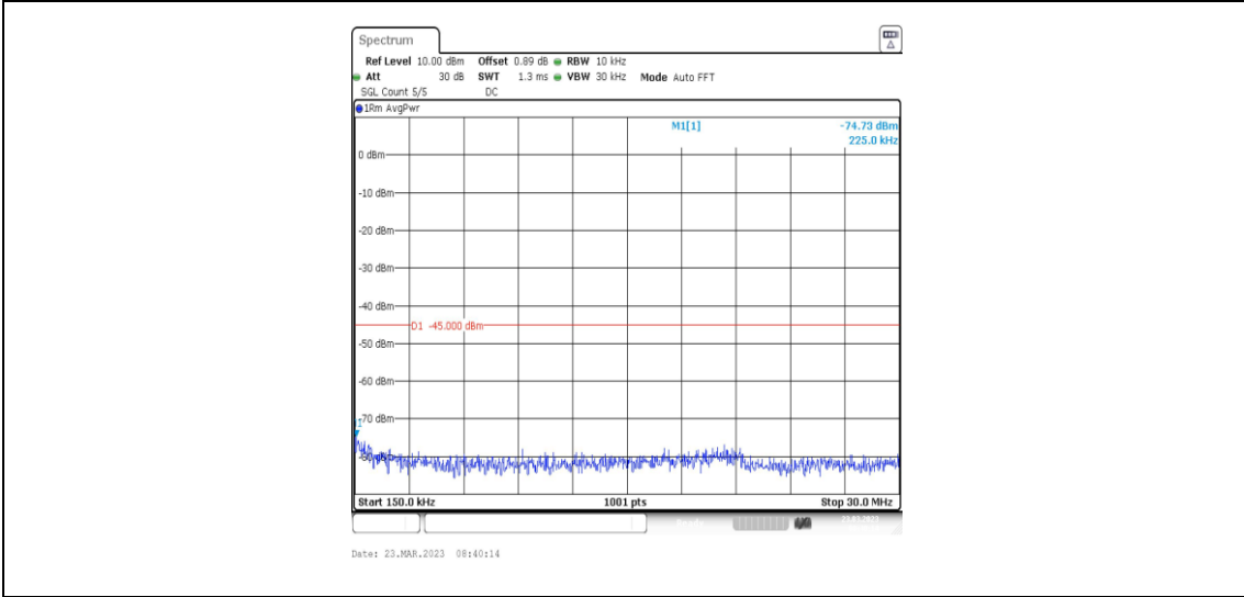
38-38-20MHz-20MHz-QPSK-QPSK-37850-38048-100RB#0-100RB#0-0.15~30MHz
