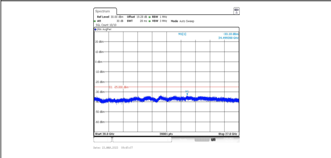
38-38-20MHz-20MHz-QPSK-QPSK-37901-38099-1RB#0-0RB#0-20000~27000MHz
