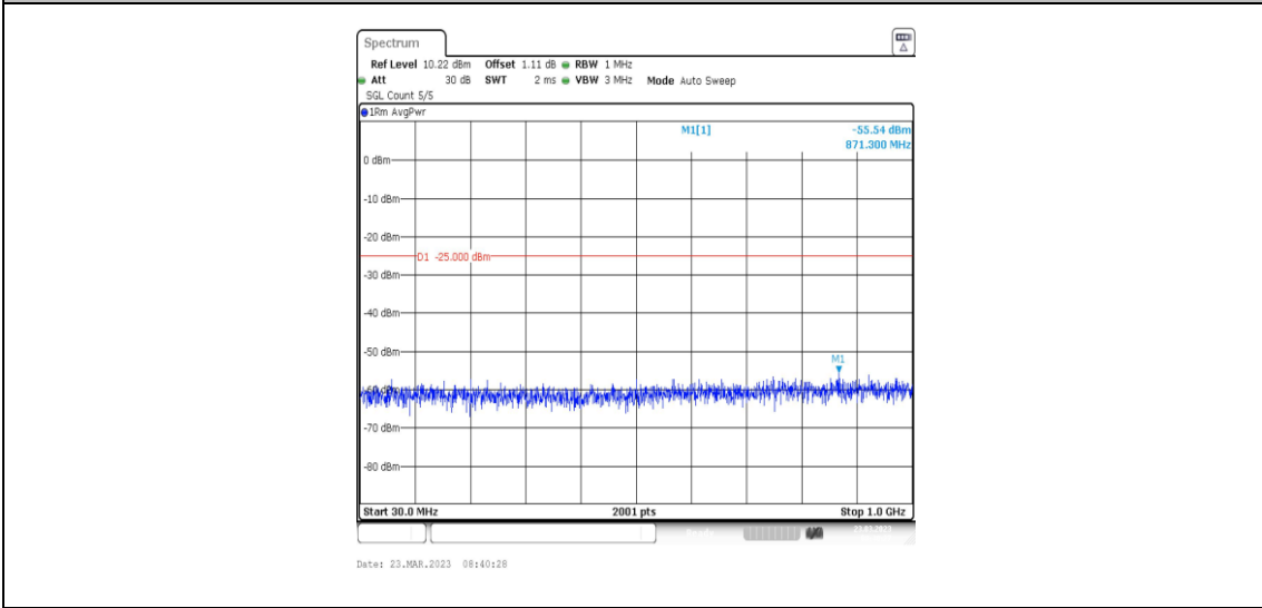
38-38-20MHz-20MHz-QPSK-QPSK-37850-38048-100RB#0-100RB#0-30~1000MHz
