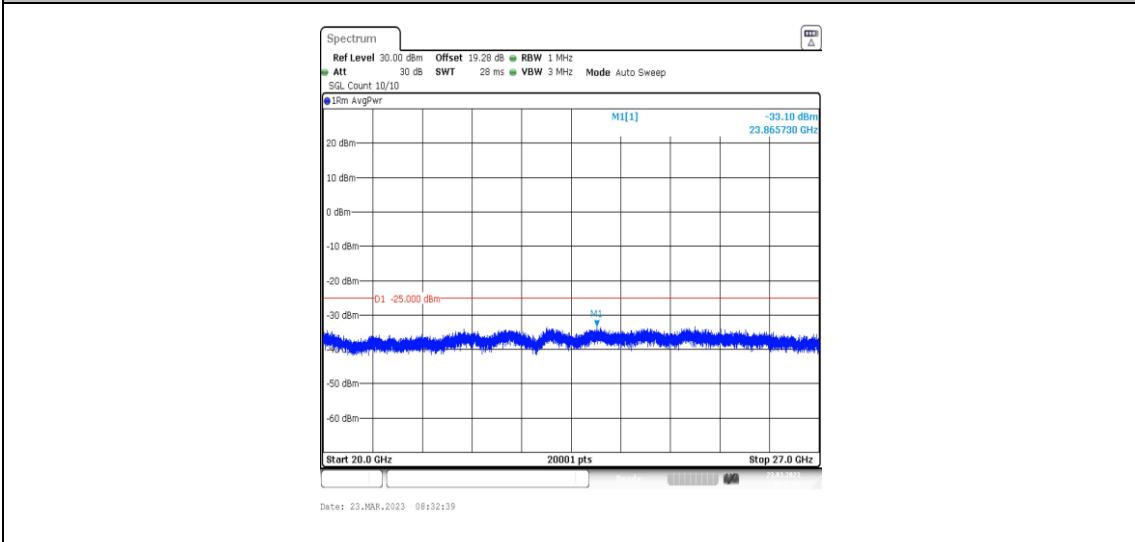
38-38-20MHz-20MHz-QPSK-QPSK-37850-38048-1RB#99-ORB#0-20000~27000MHz
