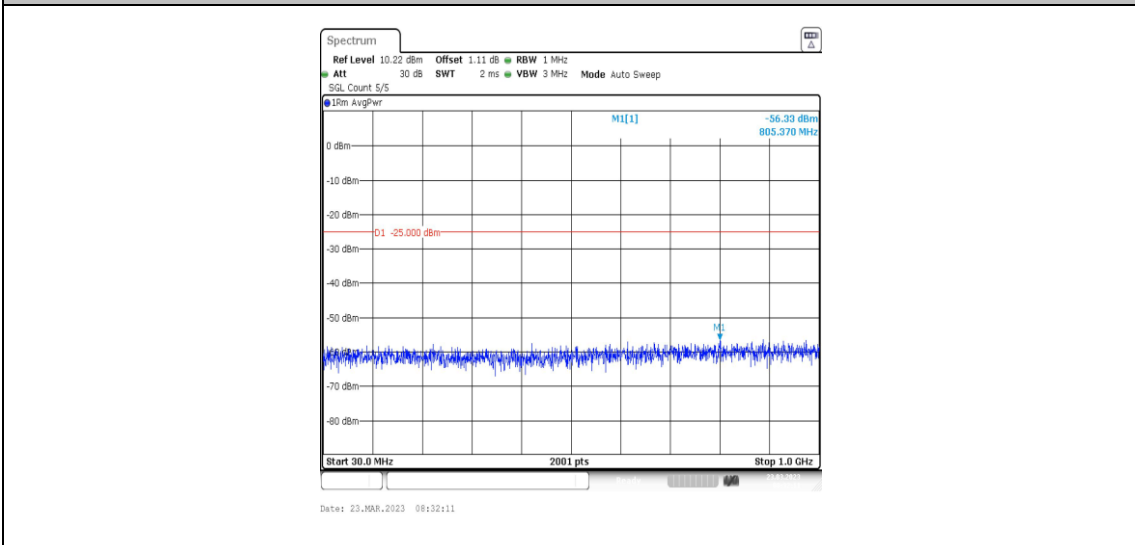
38-38-20MHz-20MHz-QPSK-QPSK-37850-38048-1RB#99-0RB#0-30~1000MHz
