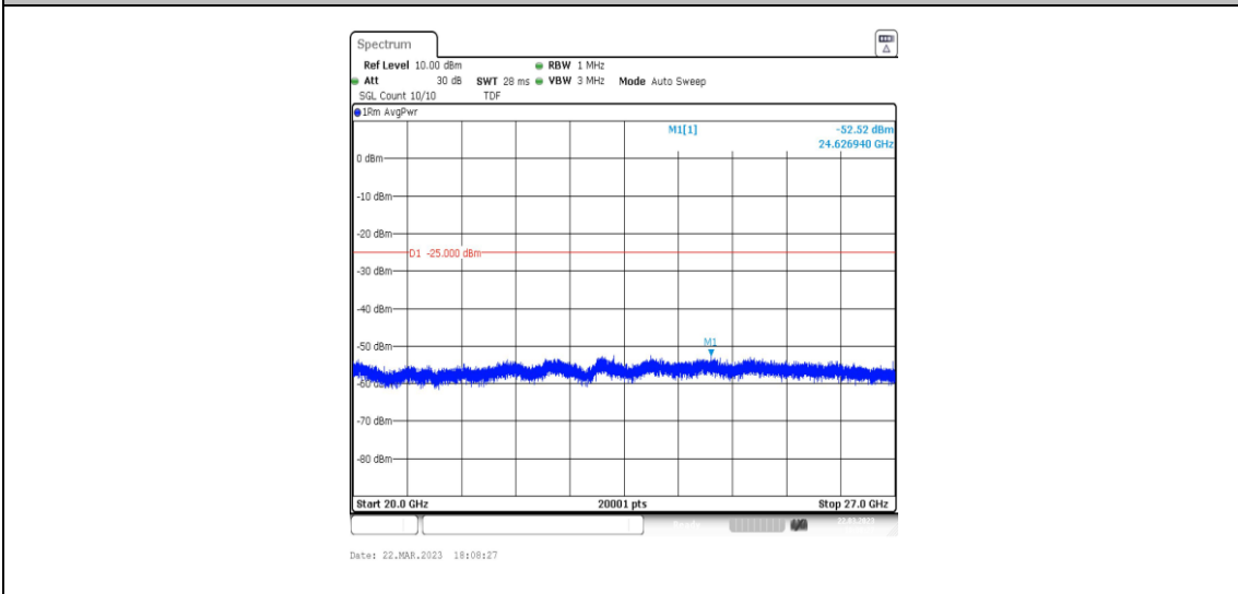
38-38-15MHz-15MHz-QPSK-QPSK-37825-37975-1RB#0-1RB#74-20000~27000MHz
