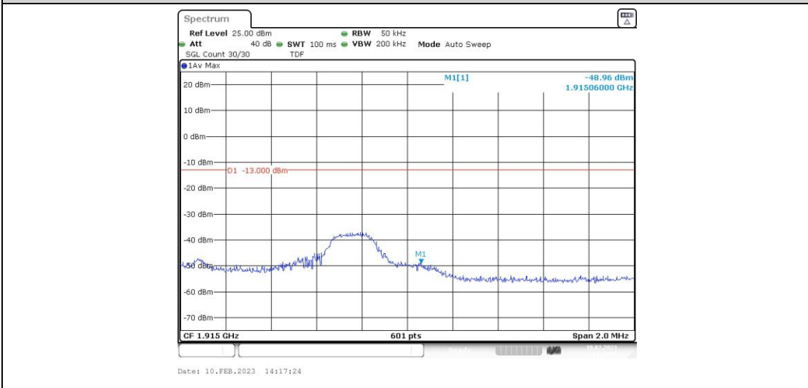
Band25-3MHz-QPSK-26675-1RB#14
