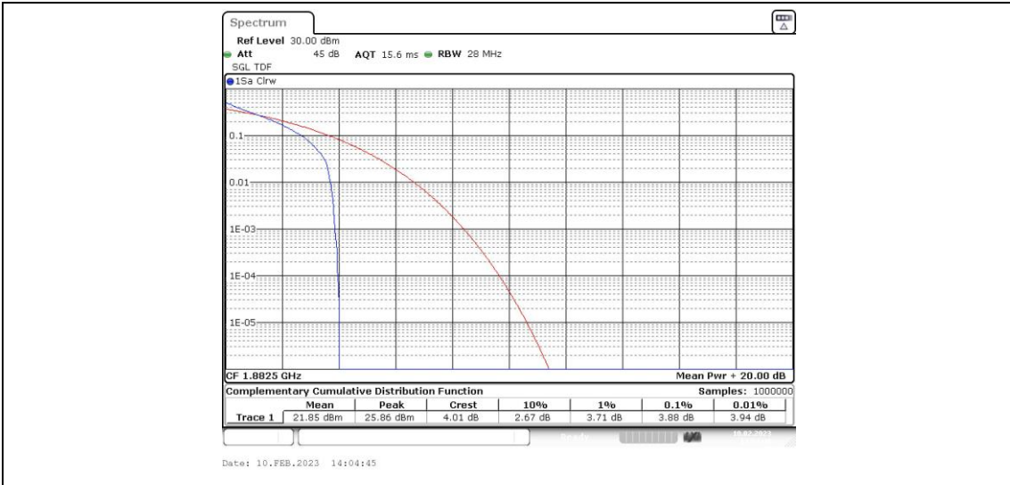
Band25-1.4MHz-QPSK-26365-6RB#0
