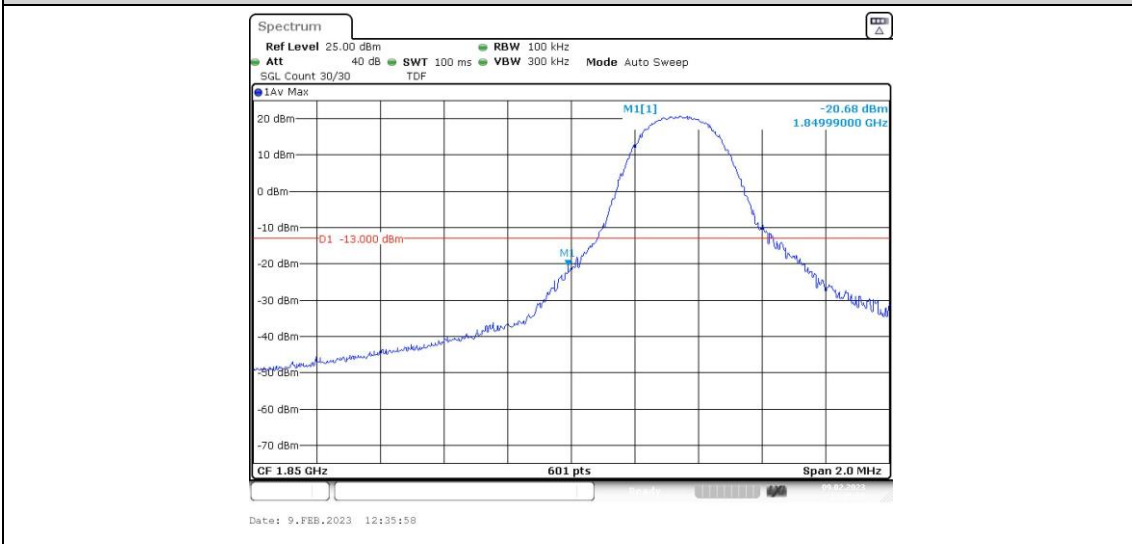
Band2-5MHz-QPSK-18625-1RB#24
