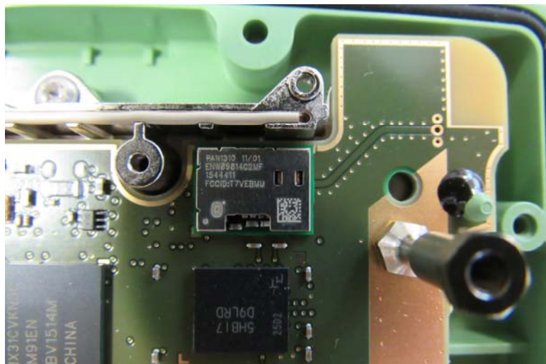
BT Module
