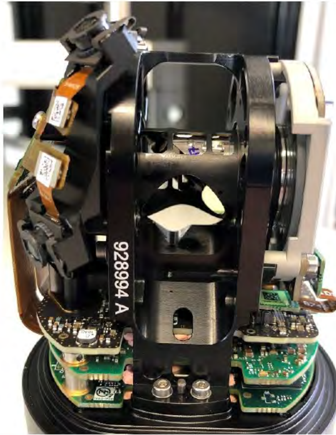
Subassembly-Lidar_FronView_Mirror
