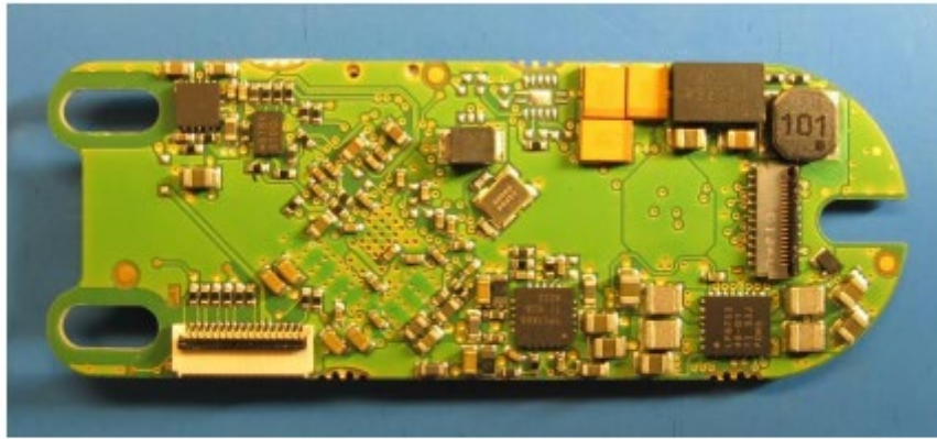
880870_Slave_Radar-Board_BOTTOM
