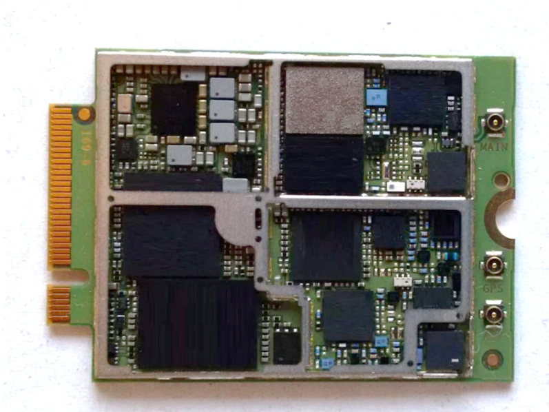
897756_LTE Bottom
