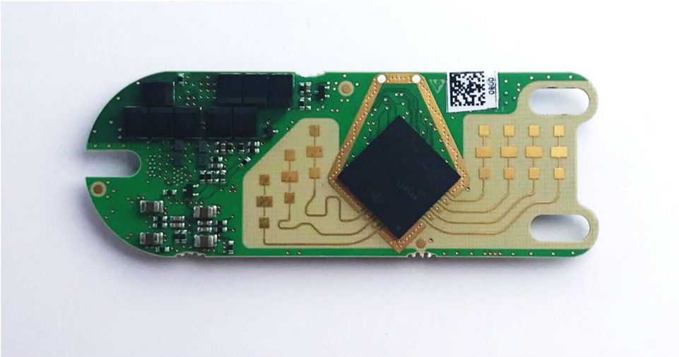
880870_Slave_Radar-Board_BOTTOM
