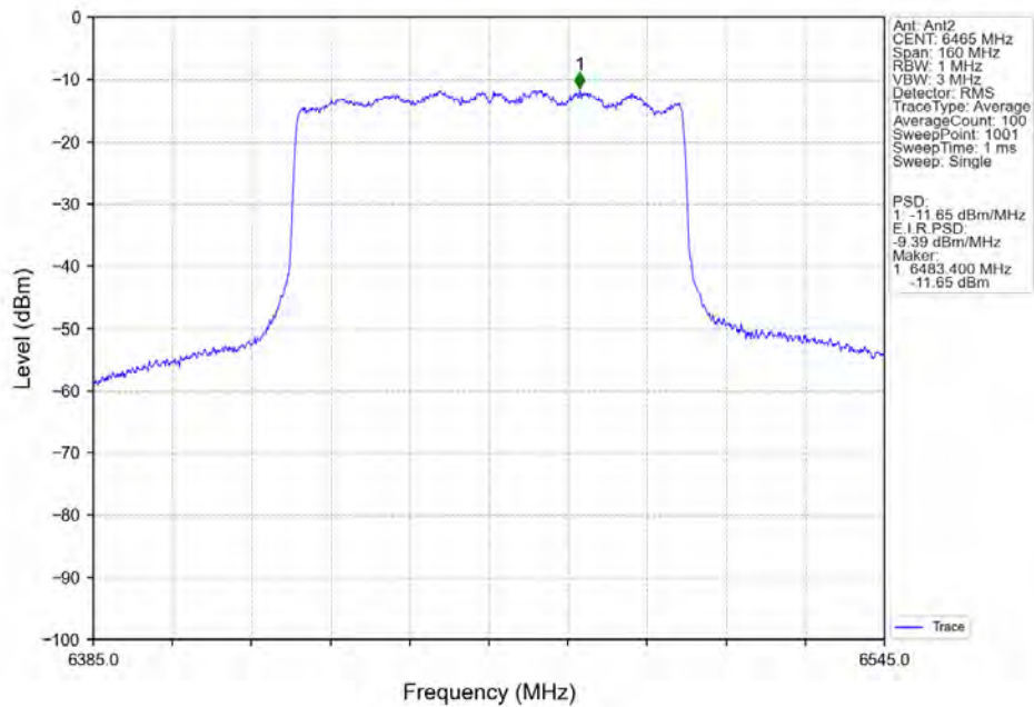
802.11ax(HEW80)_LCH_6465MHz_RU996_Left_MIMO_NTNV
