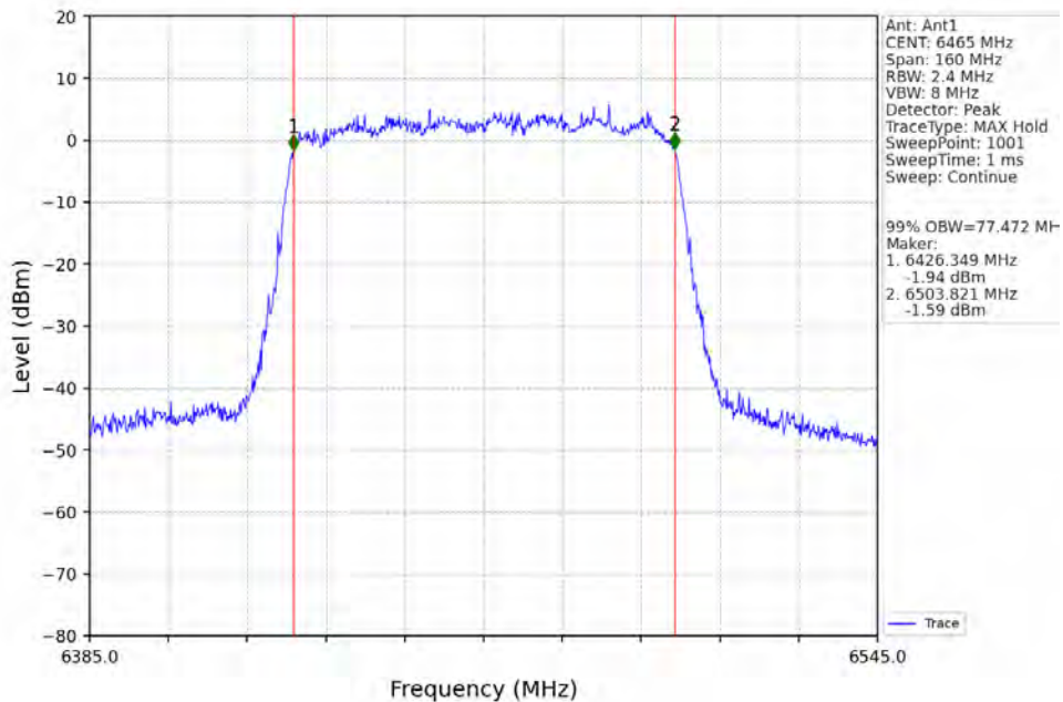
802.11ax(HEW80)_LCH_6465MHz_RU996_Left_Ant1_NTNV
