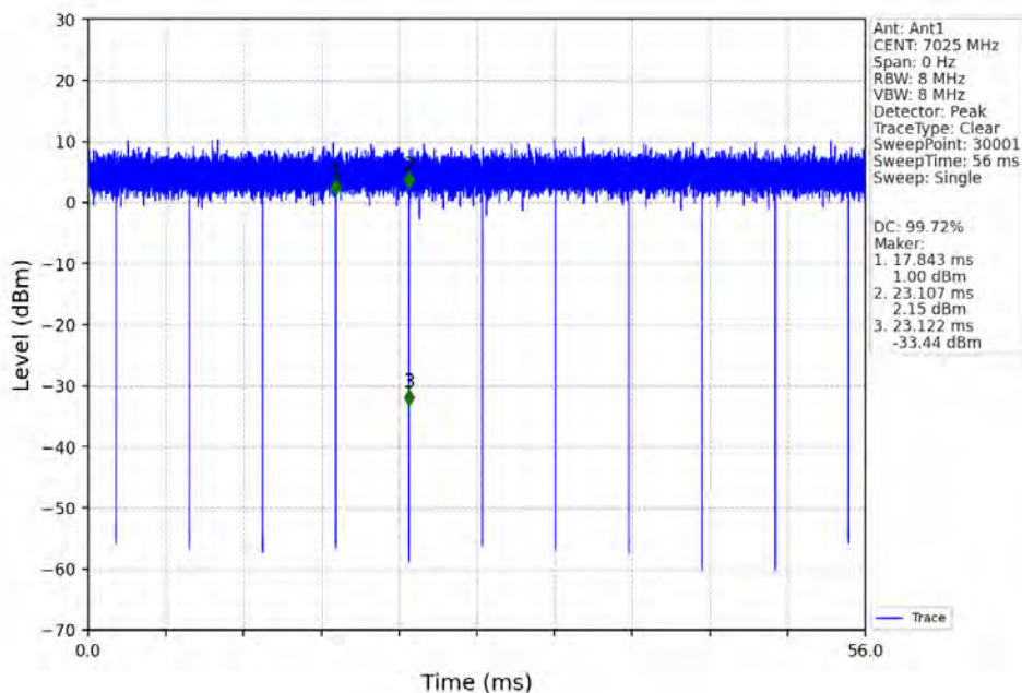
802.11ax(HEW80)_HCH_7025MHz_RU996_Left_Ant1_NTNV
