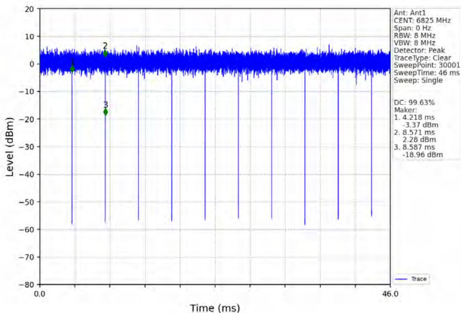
802.11ax(HEW160)_HCH_6825MHz_2xRU996_Left_Ant1_NTNV
