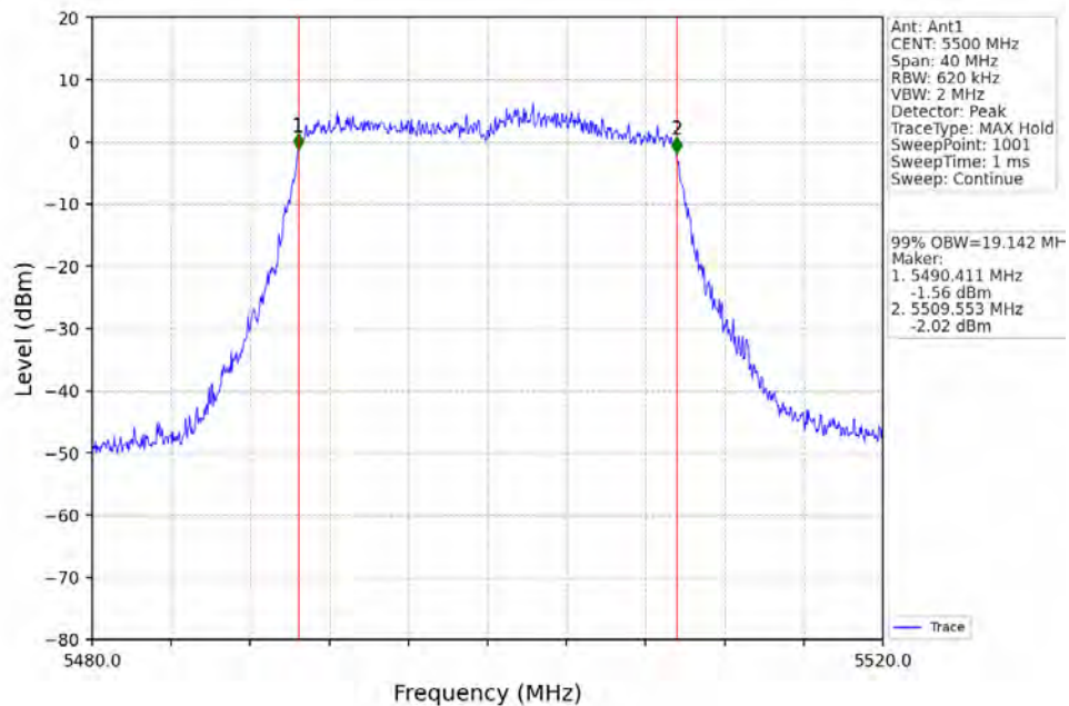
802.11ax(HEW20)_LCH_5500MHz_RU242_Left_Ant1_NTNV
