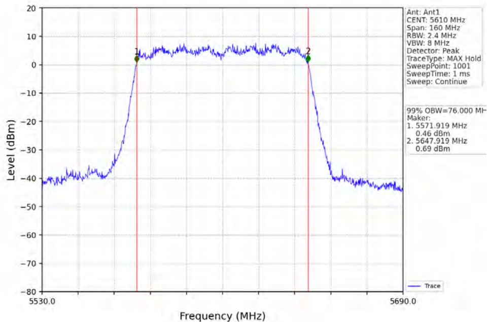
802.11ac(VHT80)_HCH_5610MHz_Ant1_NTNV
