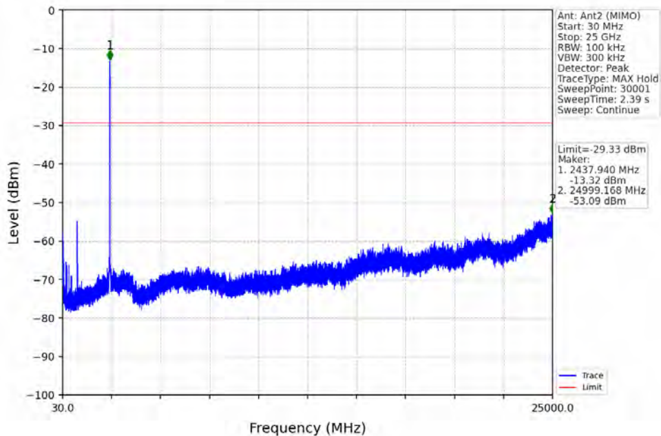
802.11ax(HEW40)_MCH_2437MHz_RU484_Left_Ant2 (MIMO)_NTNV
