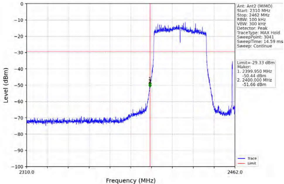
802.11ax(HEW40)_LCH_2422MHz_RU484_Left_Ant2 (MIMO)_NTNV
