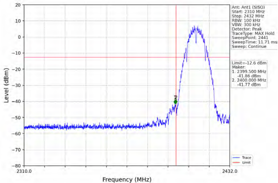
802.11b_LCH_2412MHz_Ant1 (SISO)_NTNV
