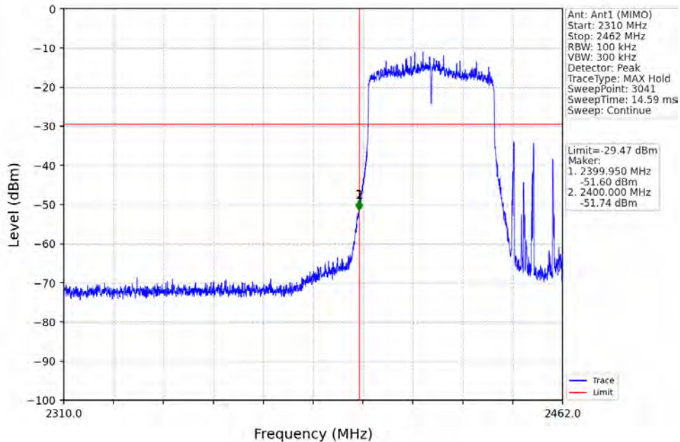
802.11ax(HEW40)_LCH_2422MHz_RU484_Left_Ant1 (MIMO)_NTNV
