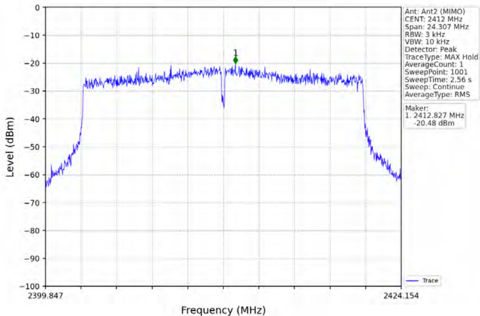
802.11ax(HEW20)_LCH_2412MHz_RU242_Left_Ant2 (MIMO)_NTNV
