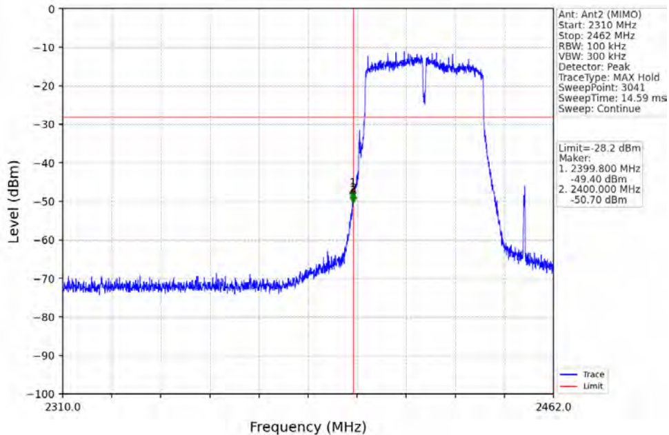
802.11n(HT40)_LCH_2422MHz_Ant2 (MIMO)_NTNV
