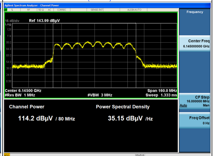
802.11ax (HE80) CDD: CH 39
