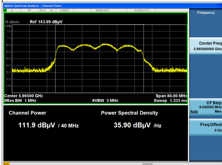
802.11ax (HE40) CDD: CH 3
