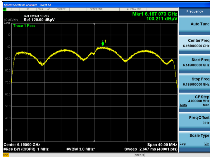
802.11ax (HE40) CDD: CH 43
