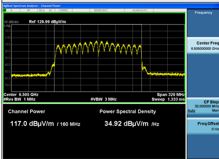
802.11ax (HE160) CDD: CH 111
