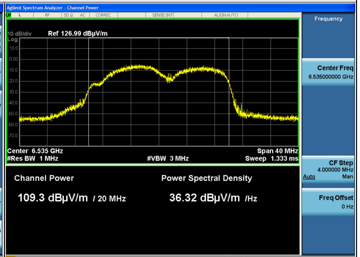
802.11ax (HE20) CDD: CH 117
