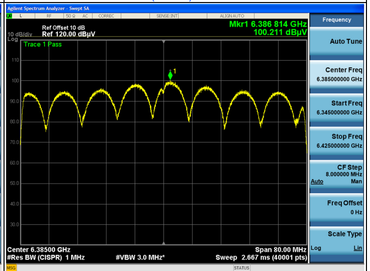
802.11ax (HE80) CDD: CH 87
