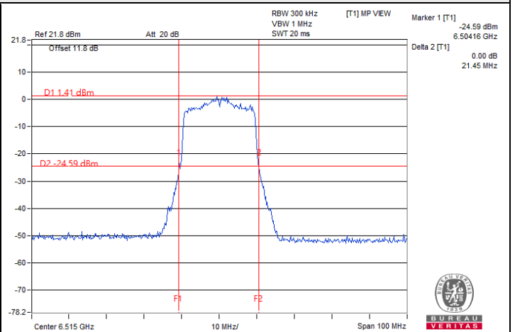
802.11ax (HE20) / Chain 1 : CH 113
