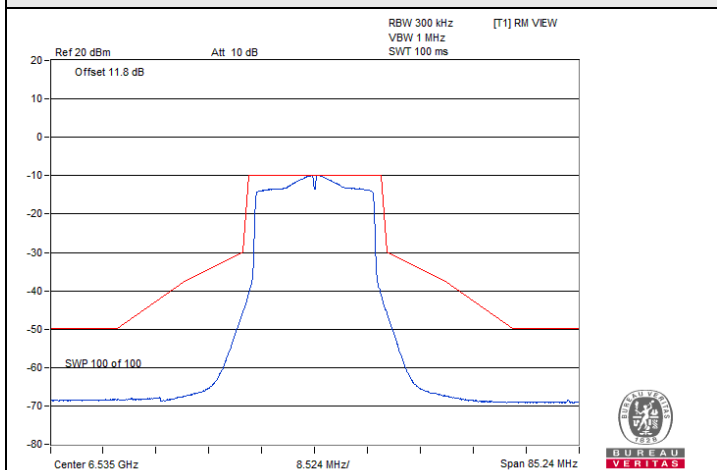
802.11ax (HE20) CDD / Chain 1 : CH 117
