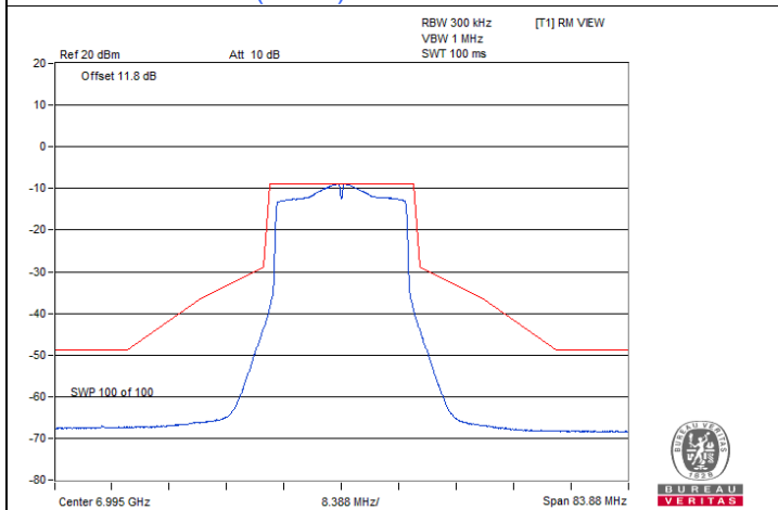
802.11ax (HE20) CDD / Chain 1 : CH 209
