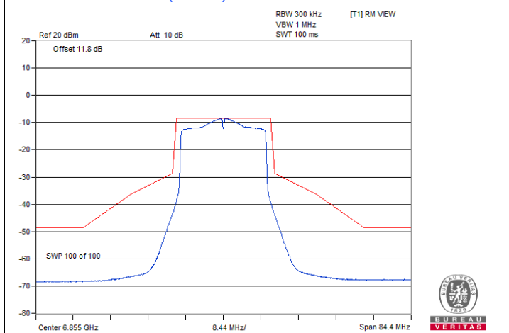
802.11ax (HE20) CDD / Chain 1 : CH 181
