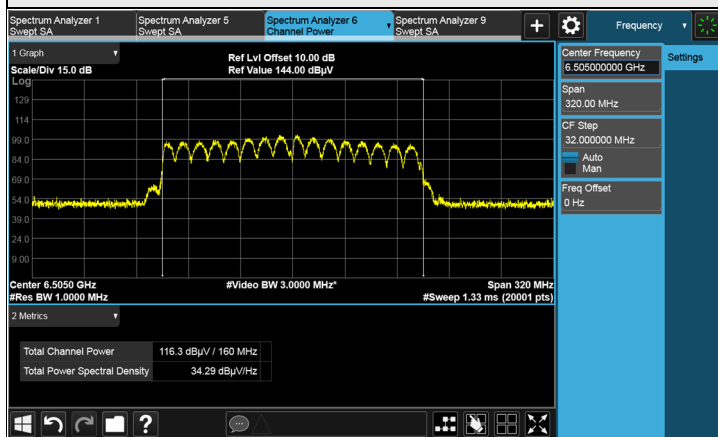
802.11ax (HE160) CDD: CH 111
