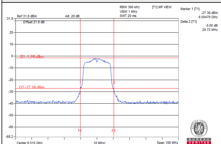
802.11a / Chain 0 : CH 113
