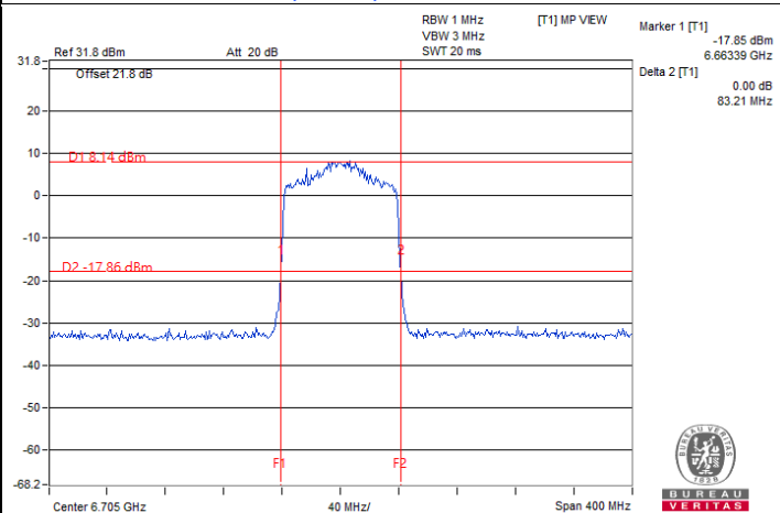
802.11ax (HE80) / Chain 0 : CH 151
