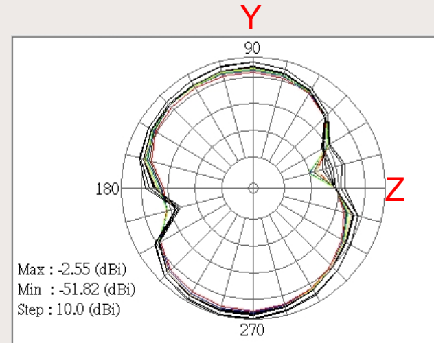
E2 plane
