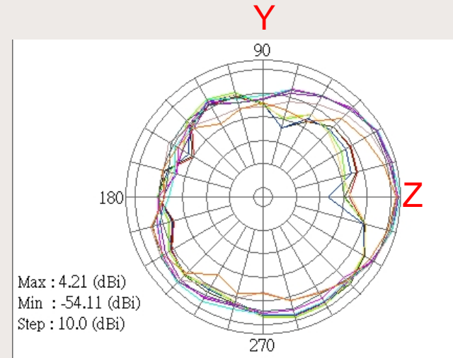
E2 plane
