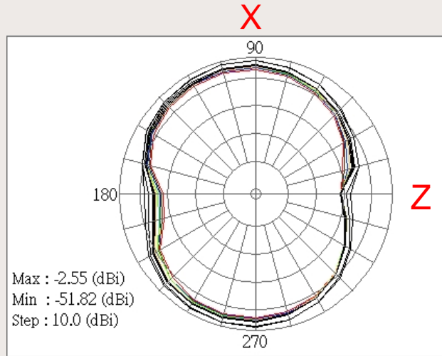
E1 plane
