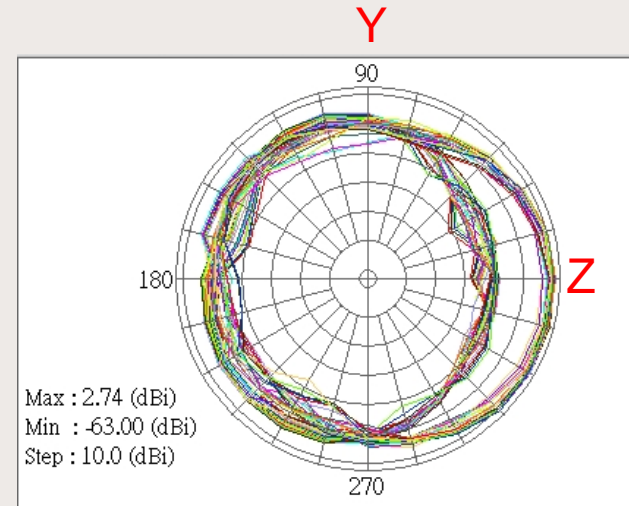
E2 plane
