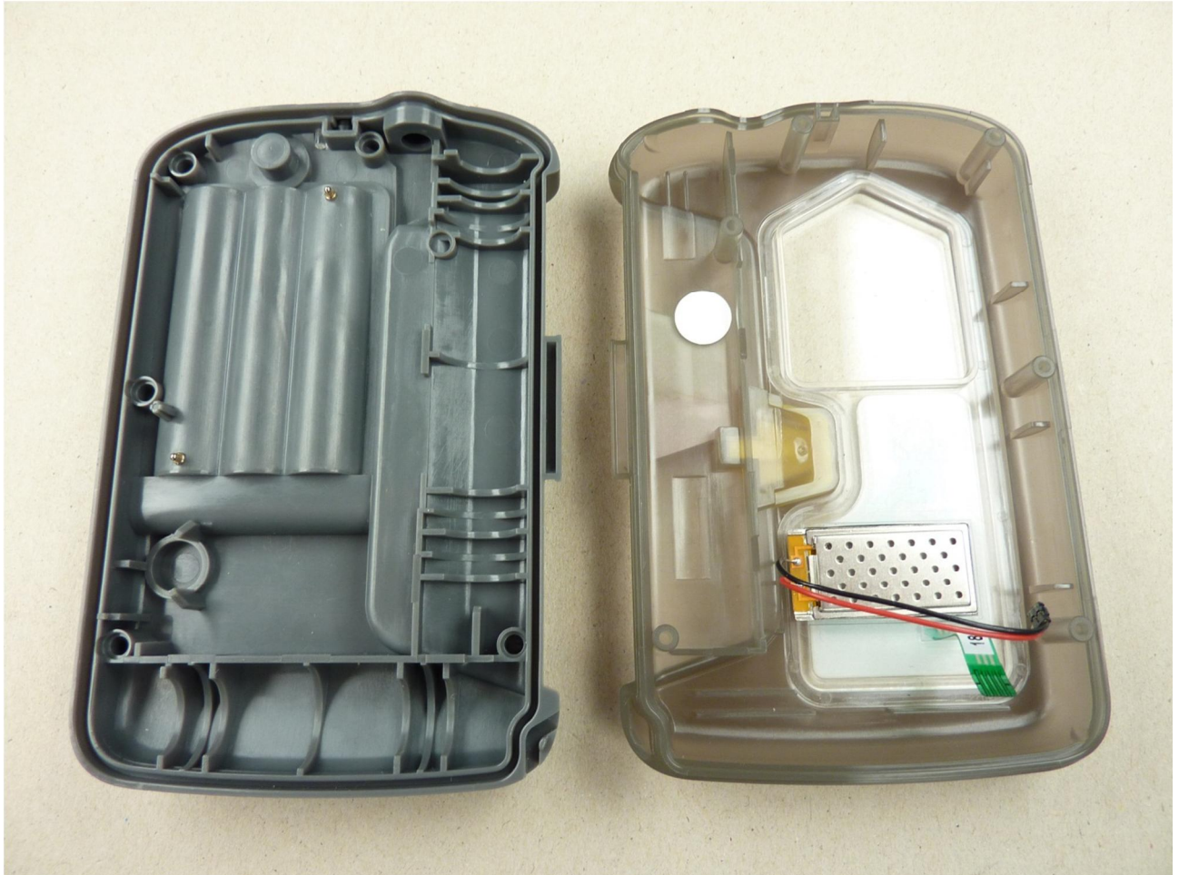
131845eut2.JPG: EUT, internal-view
