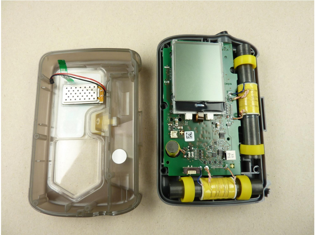
131845eut1.JPG: EUT, internal-view
