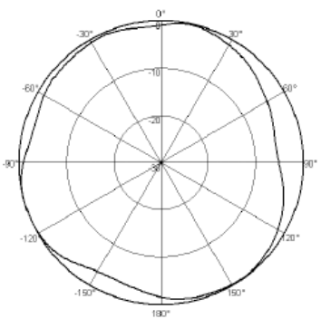
H-Plane Pattern
