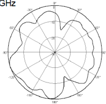
H-Plane Pattern
