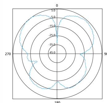
E-Plane 2.45 GHz
