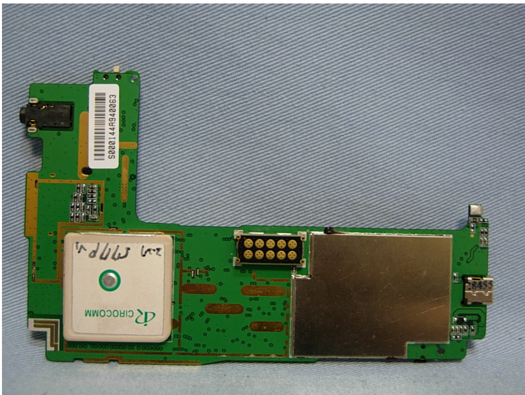
(16) EUT Photo (GPS Antenna : CIROCOMM-03A54B690011120)
