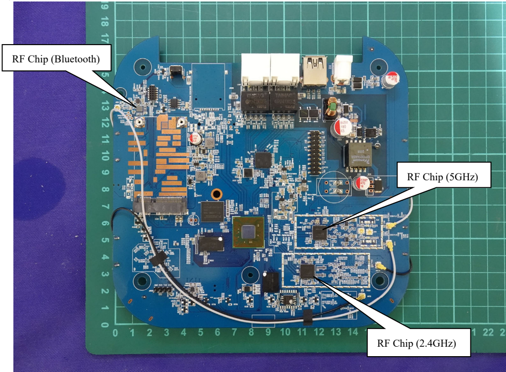
(13) EUT Photo
